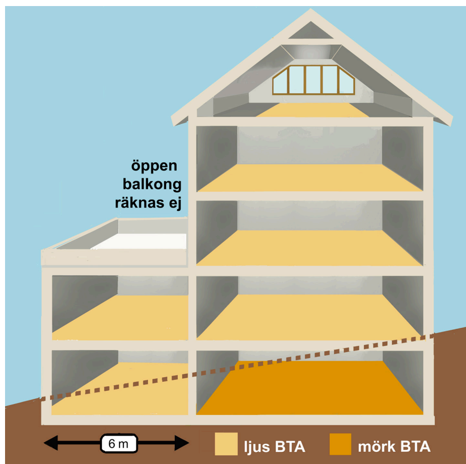
BTA-beräkning, alternativ med suterrängsvåning
