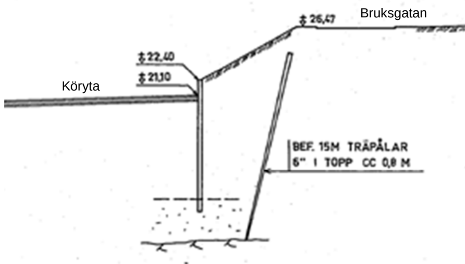
Figur 2 Sektion från sponstritning, ritning finns i bilaga 1.
