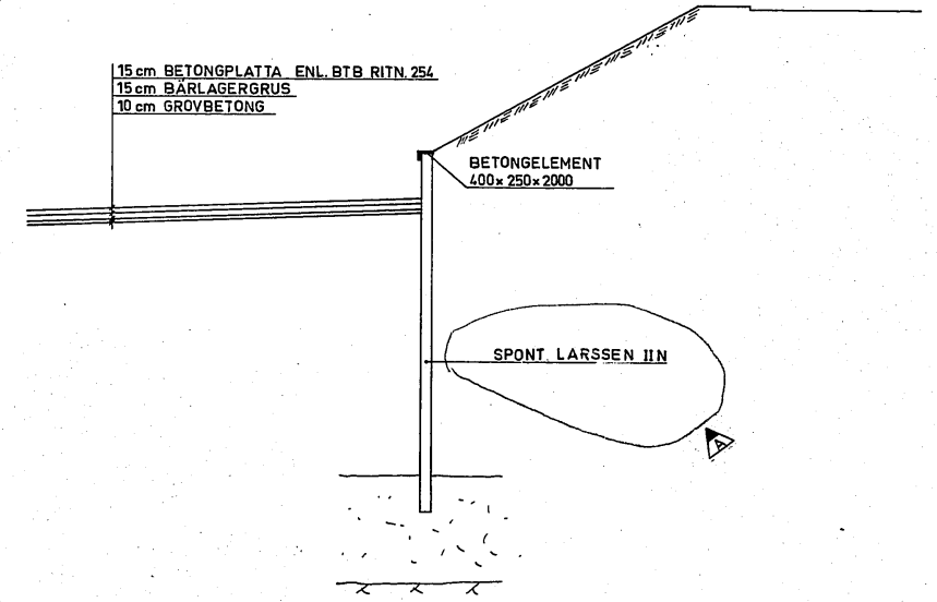
DETALJ SKALA 1:100
