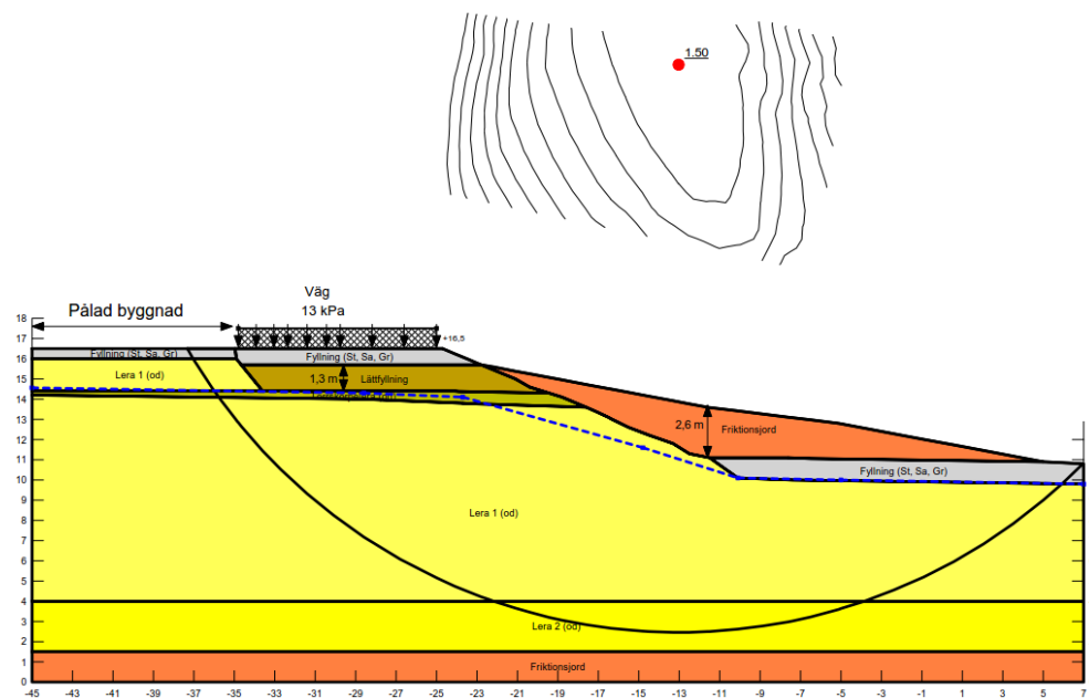
Figur 12 Åtgärdsförslag med tryckbank, sektion B odränerad analys.
