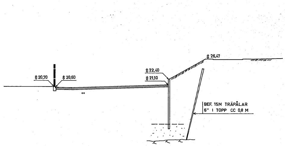
SEKTION SKALA 1:200
