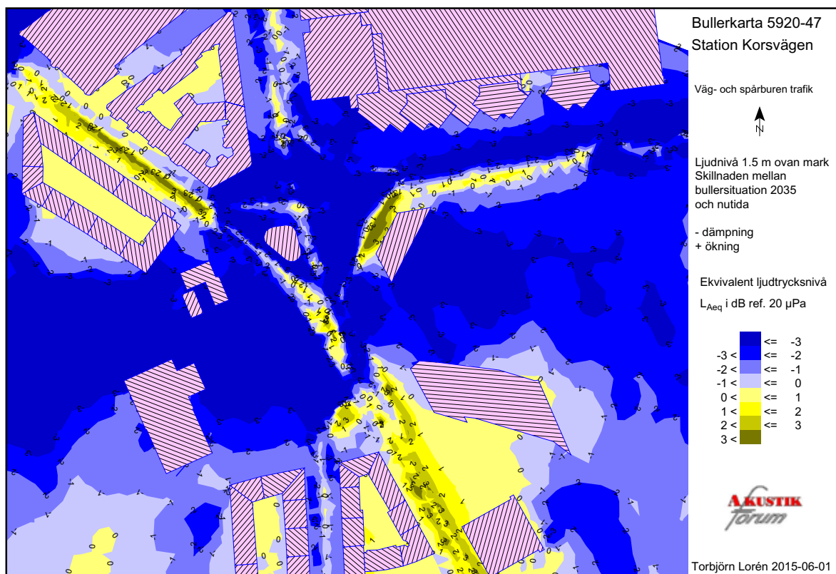
Figur 16.4.1. Skillnaden mellan bullersituation 2035 och nuläge 1,5 m ovan mark, ekvivalent ljudtrycksnivå, väg- och spårburen trafik (Akustikforum 2015-06-01)
