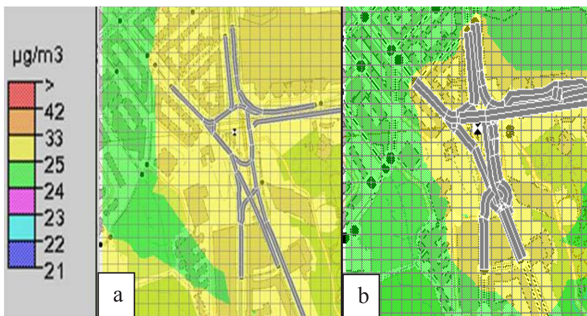
Figur 16.2.1.1 98-percentil-dygnsmedelvärdet av NO 2 -halter på Korsvägen beräknades med hjälp av Simair-korsning. a) Nollalternativ; b) Planalternativet, från Miljöförvaltnings rapport 2015:3, Beräkningar av halterna av PM10 och NO 2 i närheten av Västlänkens stationslägen under drifttid
