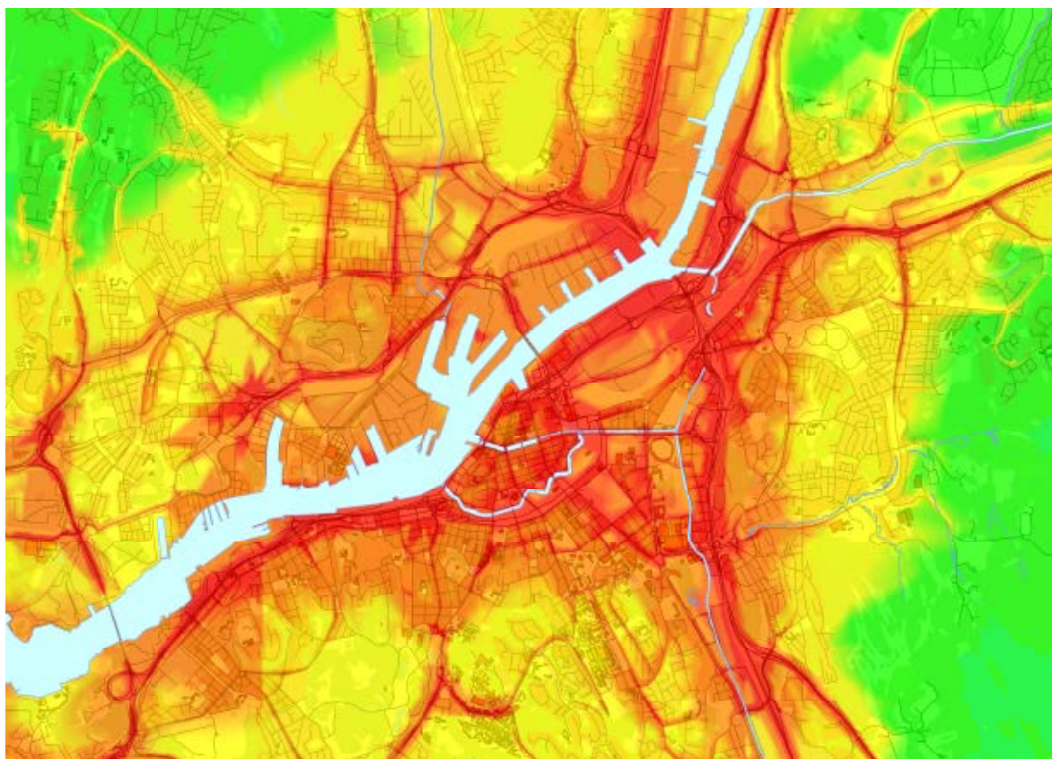
Figur 16.1.2 .Spridningskarta för 8:e högsta dygnet (år 2013) för kvävedioxid över Göteborg (utdrag från Göteborgs Stad, Miljöförvaltningen web 2015-09-08)
