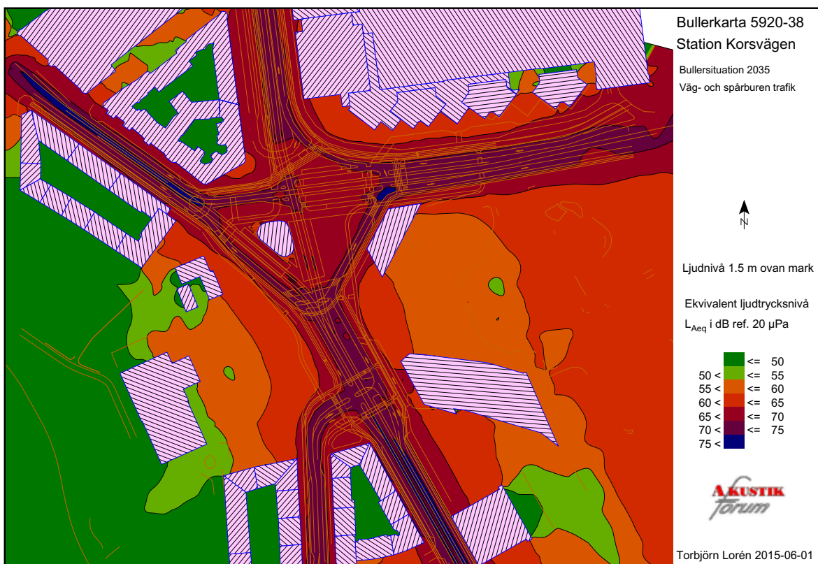
Figur 16.2.2.1. Ekvivalent ljudnivå från väg- och spårtrafik vid genomförd plan år 2035 (utdrag från Akustikforum, 2015-06-01)
