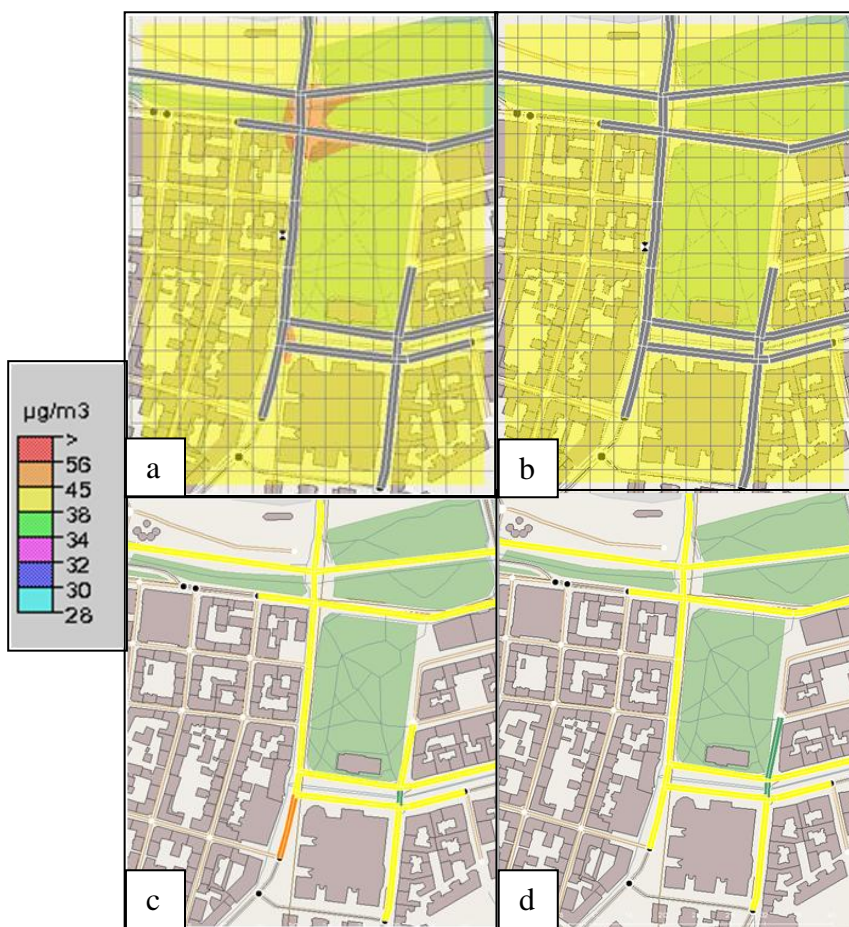
Figur 3: 98-percentil-timmedelvärde av NO 2 -halter på Haga beräknades med hjälp av Simair-korsning och Simair-väg. a) Utan Västlänken (Simair-korsning); b) Med Västlänken (Simair-korsning); c) Utan Västlänken (Simair-väg); d) Med Västlänken (Simair-väg). Svart-vit cirkel i a) och b) indikerar receptorpunkten.
