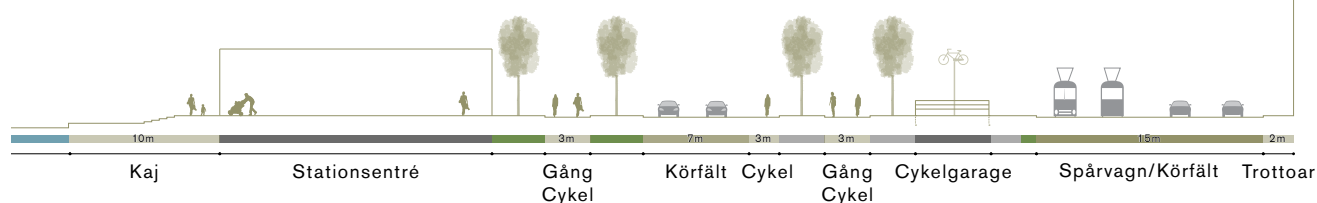
PUSTERVIKSPLATSEN SEKTION B-B' (sektionens placering på sida 34)
