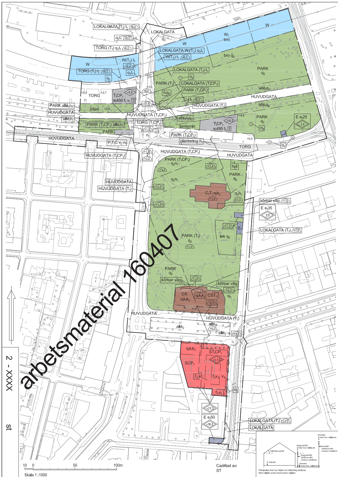
Figur 20.1:1 Planförslag för detaljplan för Station Haga.
