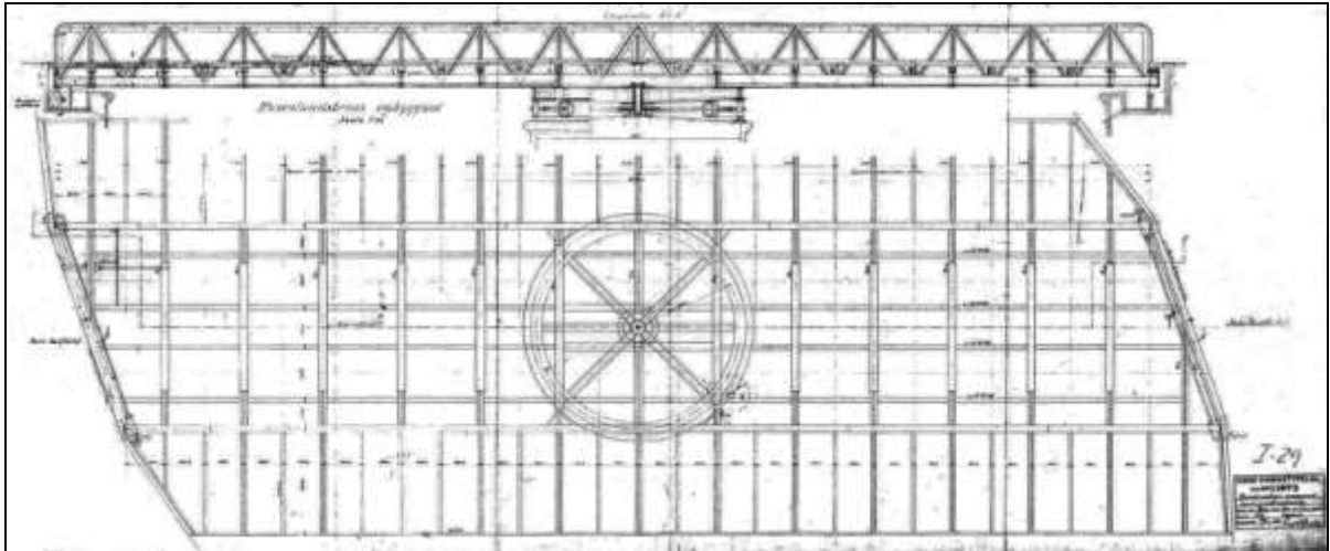
Göteborgs Hamnstyrelses ritning 1920 med sidovy och plan till nya Rosenlundsbron. Vid broöppning vrids svängspannet medurs. Ritning på Trafikkontoret.
