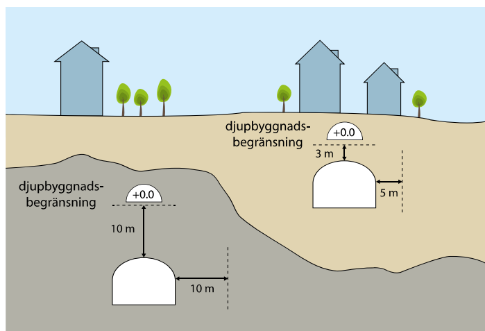
Princip som visar tunnel i berg och betongtunnel i lera samt vilket skyddsavstånd tunneln kräver.
