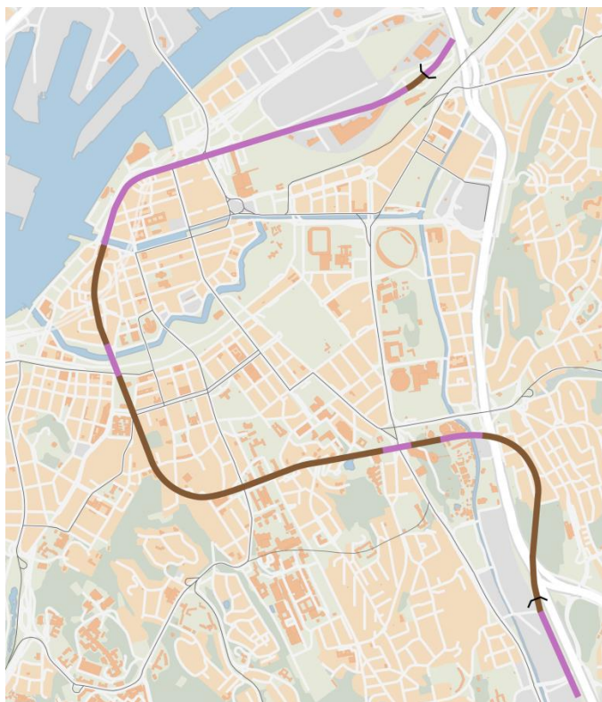
Bilden visar var tunneln går i berg (brunt) och var den går i lera/jord (rosa).
