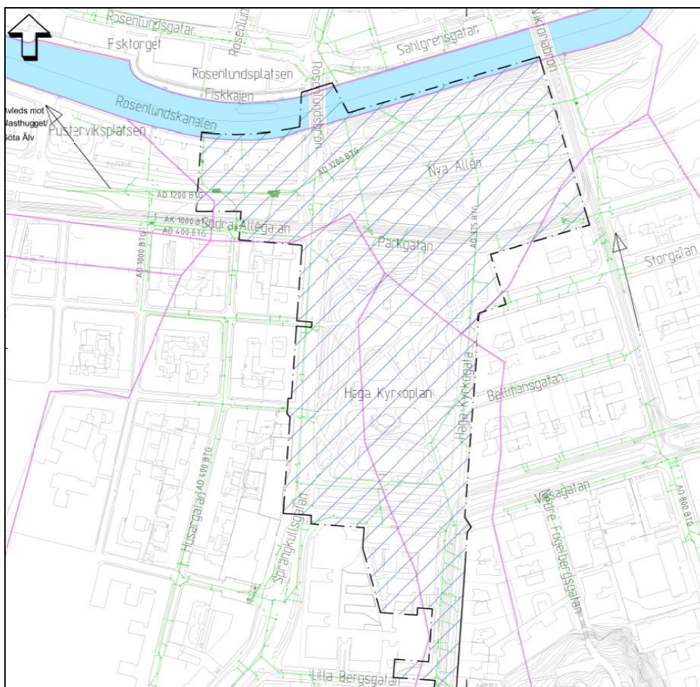
Figur 22. Avrinningsområde vid Station Haga
