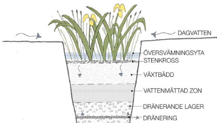
Figur 29. Uppbyggnad av en raingarden, Norconsult ©
