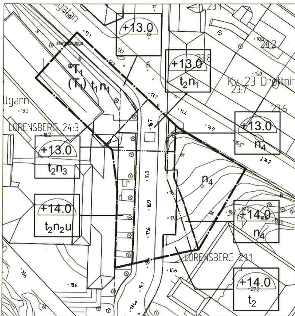
Plankarta med illustrerad gångtunnel och uppgång
