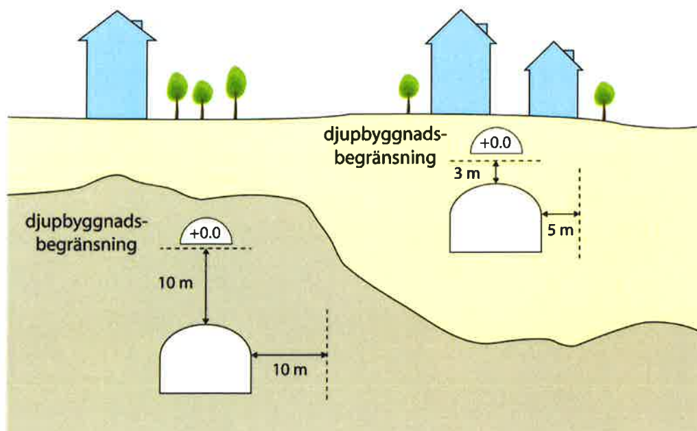
Princip som visar tunnel i berg och betongtunnel i lera med skyddsavstånd (illustration WSP).
