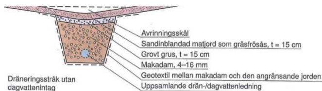
Exempel på makadamdike som täckts med växter och gräs
