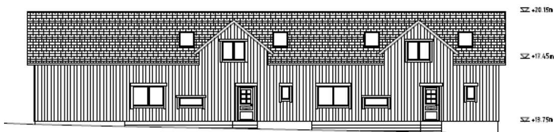
Fasad mot sydost, Vilborg Arkitekter
