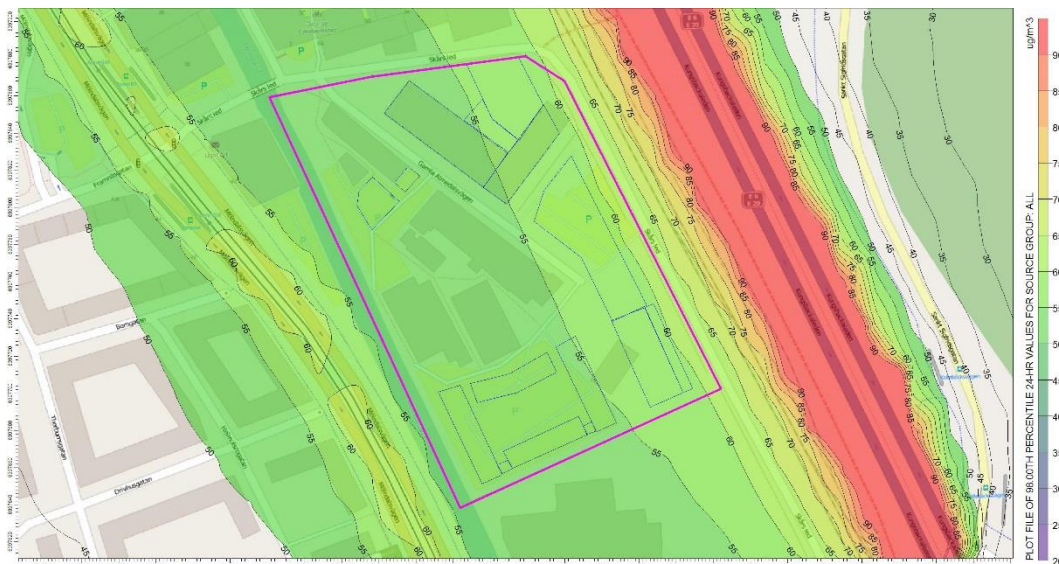
Figur 10. Framtida scenario 2020 "worst case", beräknade halter av kvävedioxid som dygnsmedelvärden. Planområdet markeras med lila linje och föreslagna byggnader med blå
