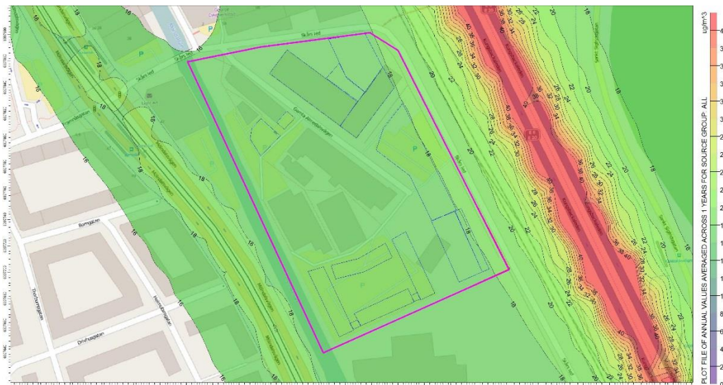
Figur 18. Framtida scenario 2020 "worst case", beräknade halter av partiklar ( PM_{10} ) som årsmedelvärden. Planområdet markeras med lila linje och föreslagna byggnader med blå
