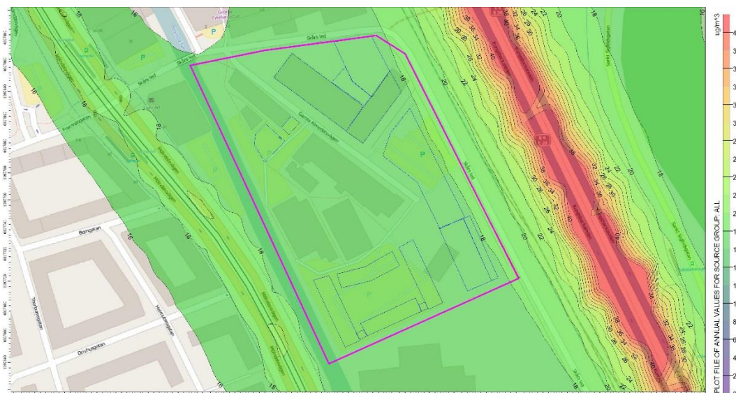
Figur 17. Framtida scenario 2020, beräknade halter av partiklar ( PM_{10} ) som årsmedelvärden. Planområdet markeras med lila linje och föreslagna byggnader med blå
