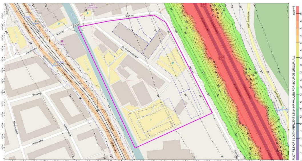
Figur 20. Nuvarande situation 2013/2015, beräknade halter av partiklar ( PM_{10} ) som dygnsmedelvärden. Planområdet markeras med lila linje och föreslagna byggnader med blå
