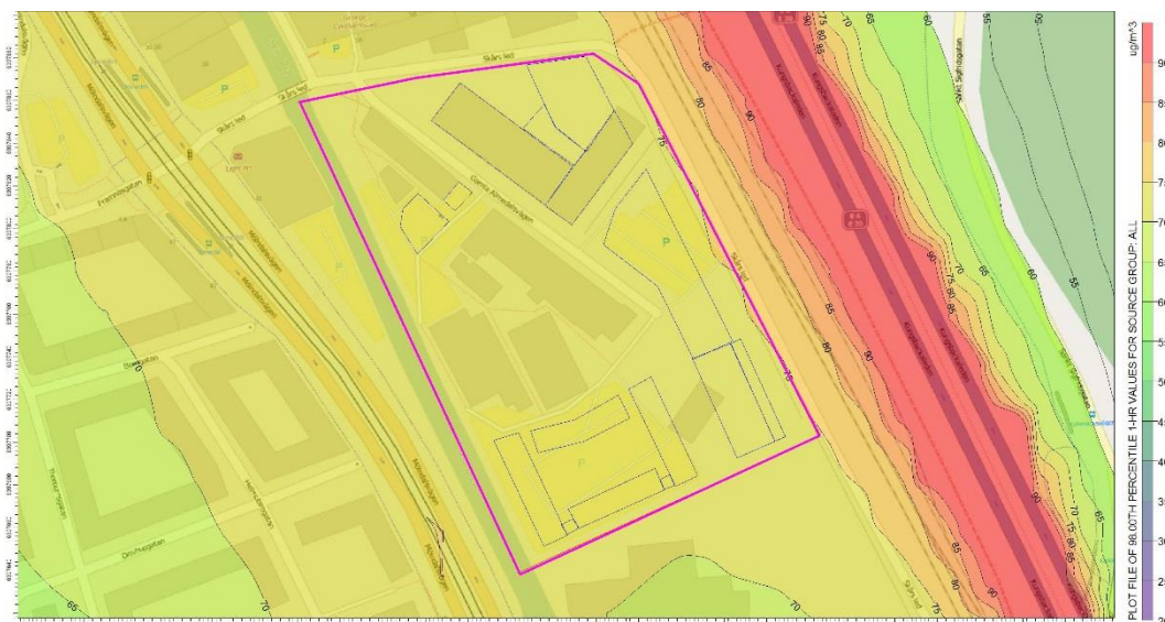
Figur 13. Framtida scenario 2020, beräknade halter av kvävedioxid som timmedelvärden. Planområdet markeras med lila linje och föreslagna byggnader med blå
