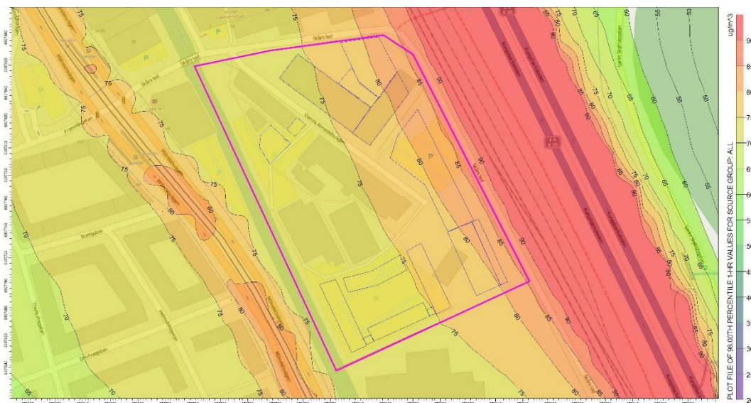
Figur 14. Framtida scenario 2020 "worst case", beräknade halter av kvävedioxid som timmedelvärden. Planområdet markeras med lila linje och föreslagna byggnader med blå
