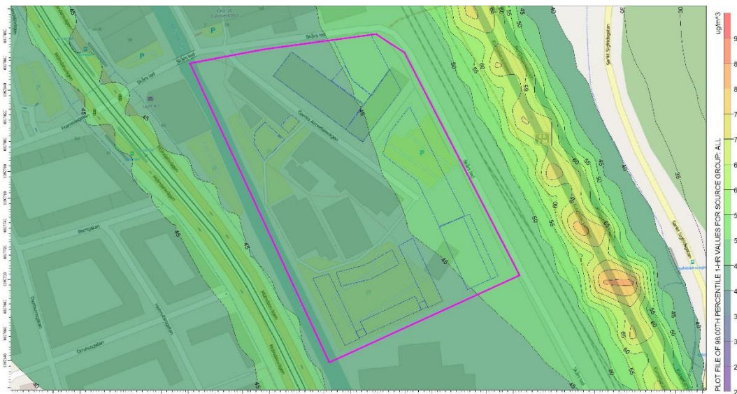
Figur 15. Framtida scenario 2030, beräknade halter av kvävedioxid som timmedelvärden. Planområdet markeras med lila linje och föreslagna byggnader med blå
