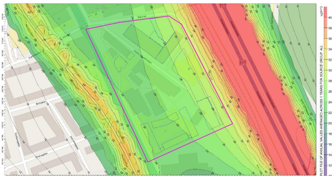
Figur 6. Framtida scenario 2020 "worst case", beräknade halter av kvävedioxid som årsmedelvärden. Planområdet markeras med lila linje och föreslagna byggnader med blå
