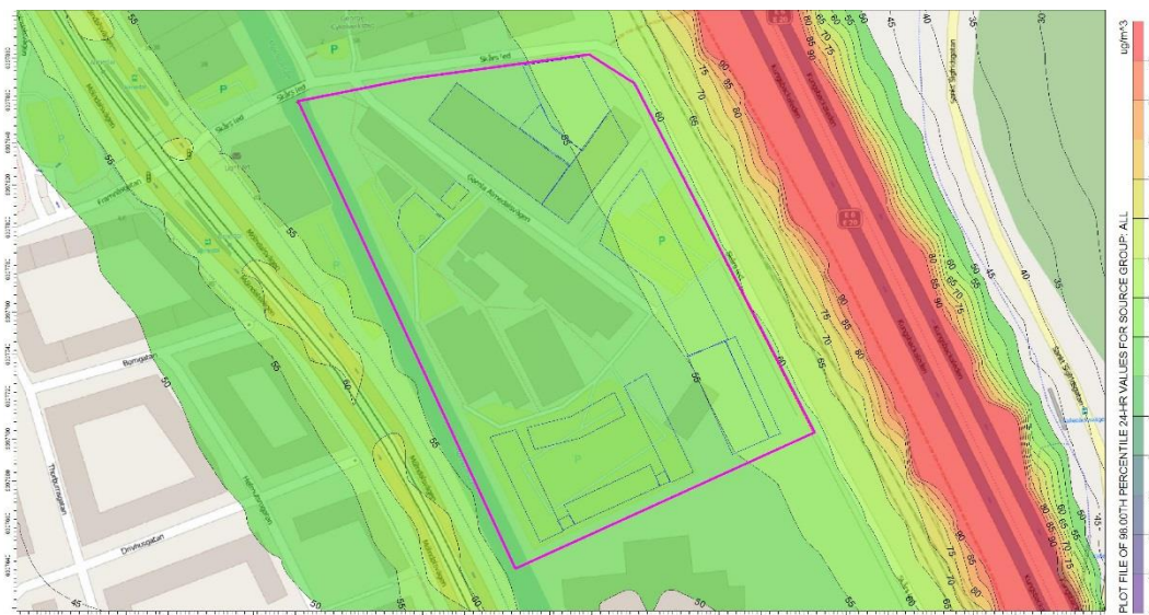
Figur 8. Nuvarande situation 2013/2015, beräknade halter av kvävedioxid som dygnsmedelvärden. Planområdet markeras med lila linje och föreslagna byggnader med blå
