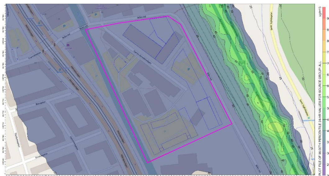
Figur 11. Framtida scenario 2030, beräknade halter av kvävedioxid som dygnsmedelvärden. Planområdet markeras med lila linje och föreslagna byggnader med blå
