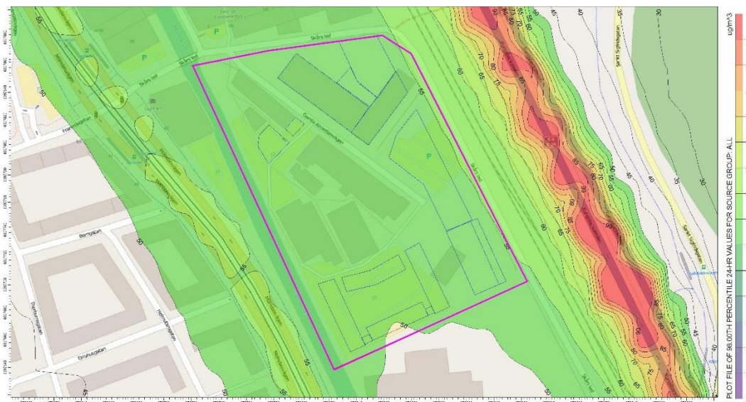
Figur 9. Framtida scenario 2020, beräknade halter av kvävedioxid som dygnsmedelvärden. Planområdet markeras med lila linje och föreslagna byggnader med blå
