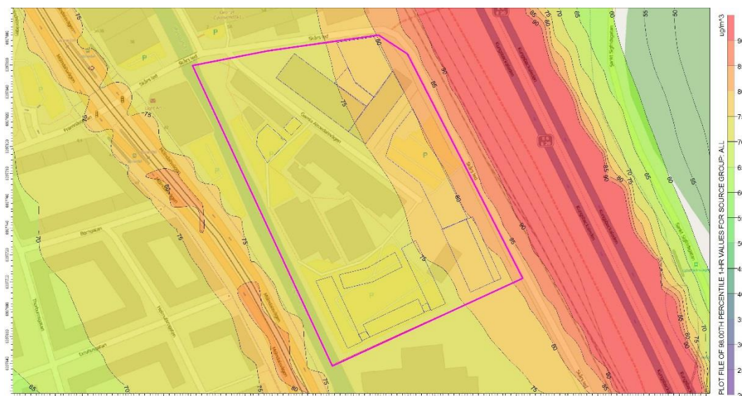
Figur 12. Nuvarande situation 2013/2015, beräknade halter av kvävedioxid som timmedelvärden. Planområdet markeras med lila linje och föreslagna byggnader med blå
