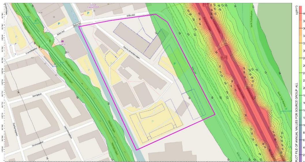
Figur 19. Framtida scenario 2030, beräknade halter av partiklar ( PM_{10} ) som årsmedelvärden. Planområdet markeras med lila linje och föreslagna byggnader med blå
