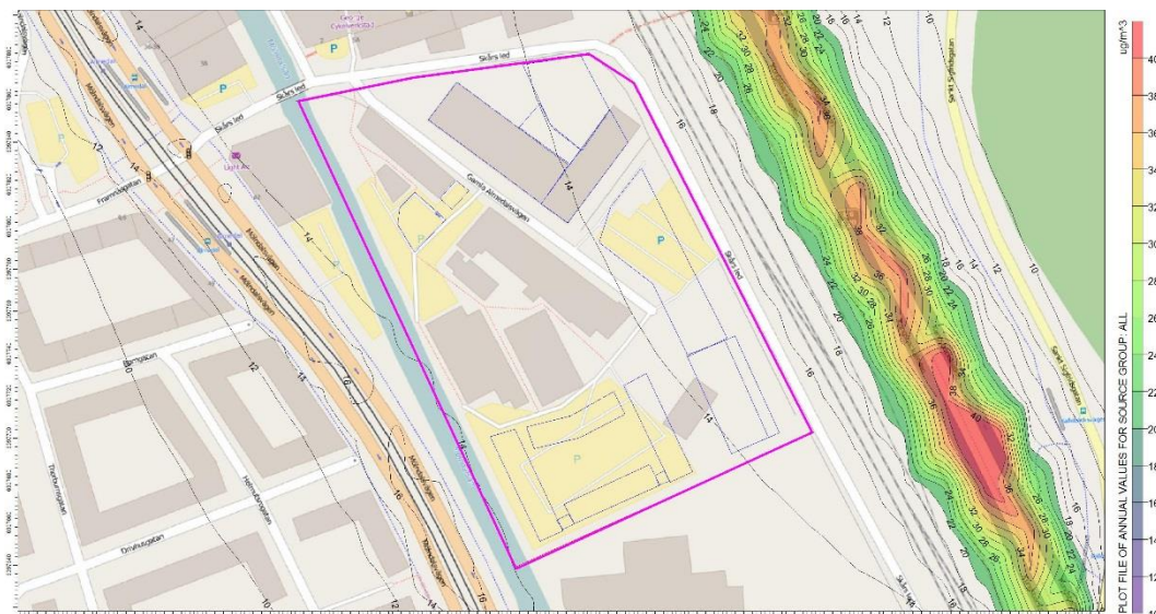
Figur 7. Framtida scenario 2030, beräknade halter av kvävedioxid som årsmedelvärden. Planområdet markeras med lila linje och föreslagna byggnader med blå
