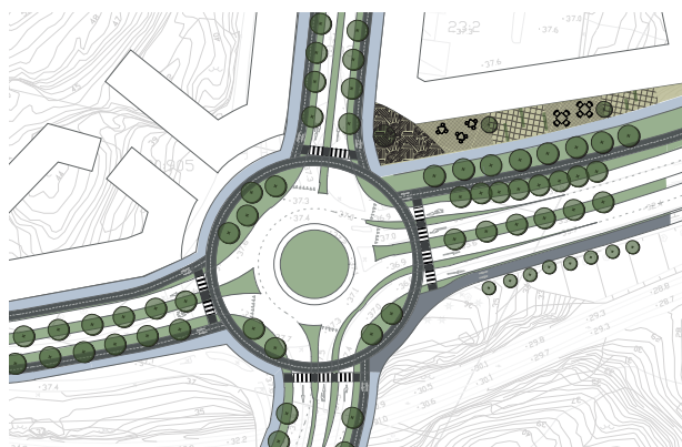
Bild: Principutformning utan extra svängfält från norr och väster.
