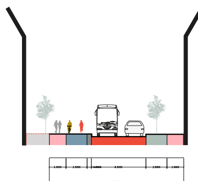
Bild: Större lokalgata. Exempel på sektion för Blidvädersgatan. Genom att flytta och bygga om gatan möjliggörs hela bostadskvarter mellan Blidvädersgatan och Yrvädersgatan. Sektionen gäller även för bussgator och huvudgator med höga cykelflöden.
