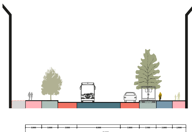
Bild: Huvudgata med separerad kollektivtrafik. Exempel på sektion över Yrvädersgatan med separata körfält för kollektivtrafik med dubbelsidig bebyggelse.
