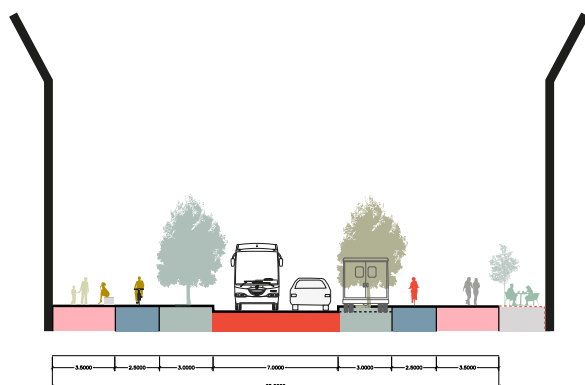
Bild: Huvudgata. Exempel på sektion för Sommarvädersgatan med dubbelsidig bebyggelse. Här kan generösa utrymmen anordnas för gående och cyklister när kollektivtrafiken inte separeras från övrig trafik. Förgårdsmark kan variera utefter sträckningen.
