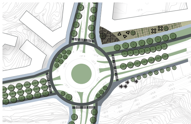
Bild: Principutformning med extra svängfält från Sommarvädersgatan och Höstvädersgatan.
