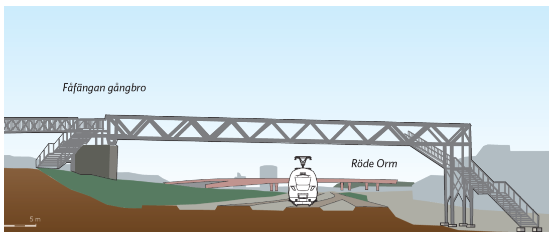
Sektion i höjd med ny gångbro vid befintlig gångbro "Fåfången" västerut. Från järnvägsplan
