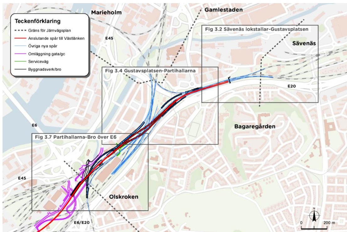
Översikt av Olskroken och de tre deletapper som beskrivs. Från järnvägsplaner.
