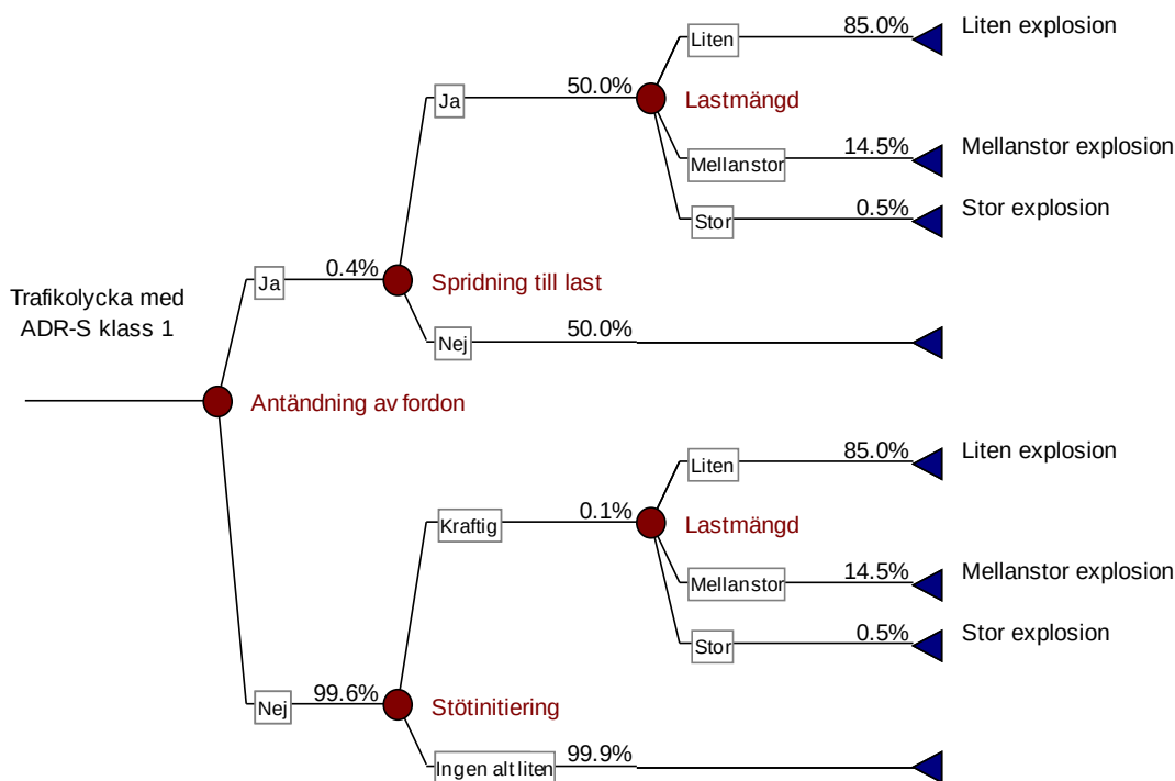
Figur 15. Händelseträd med sannolikheter för ADR-S klass 1.
