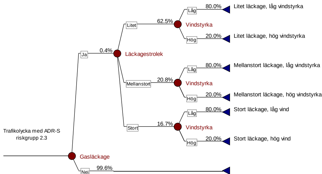
Figur 17. Händelseträd med sannolikheter för ADR-S klass 2.3.
