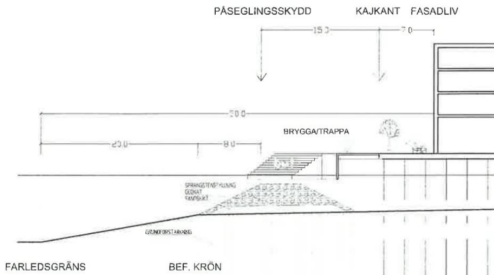
Figur 14. Typsektion avseende påseglingsskydd vid kaj (27).
