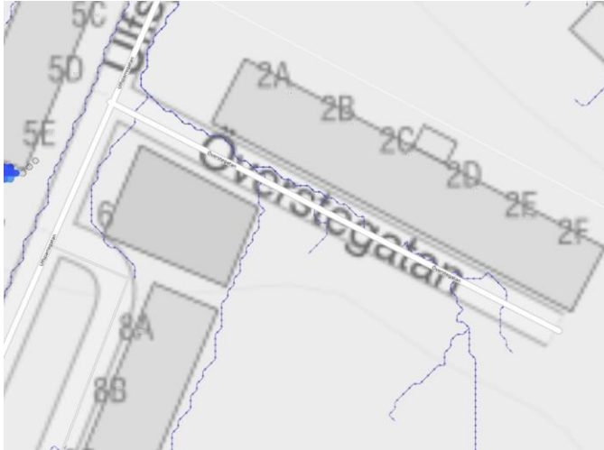
Figur 9. Resultat från lågpunktskartering med befintliga rinnvägar. Modellen har belastats med 70 mm regn. Ingen större vattensamling uppstår inom planområdet.
