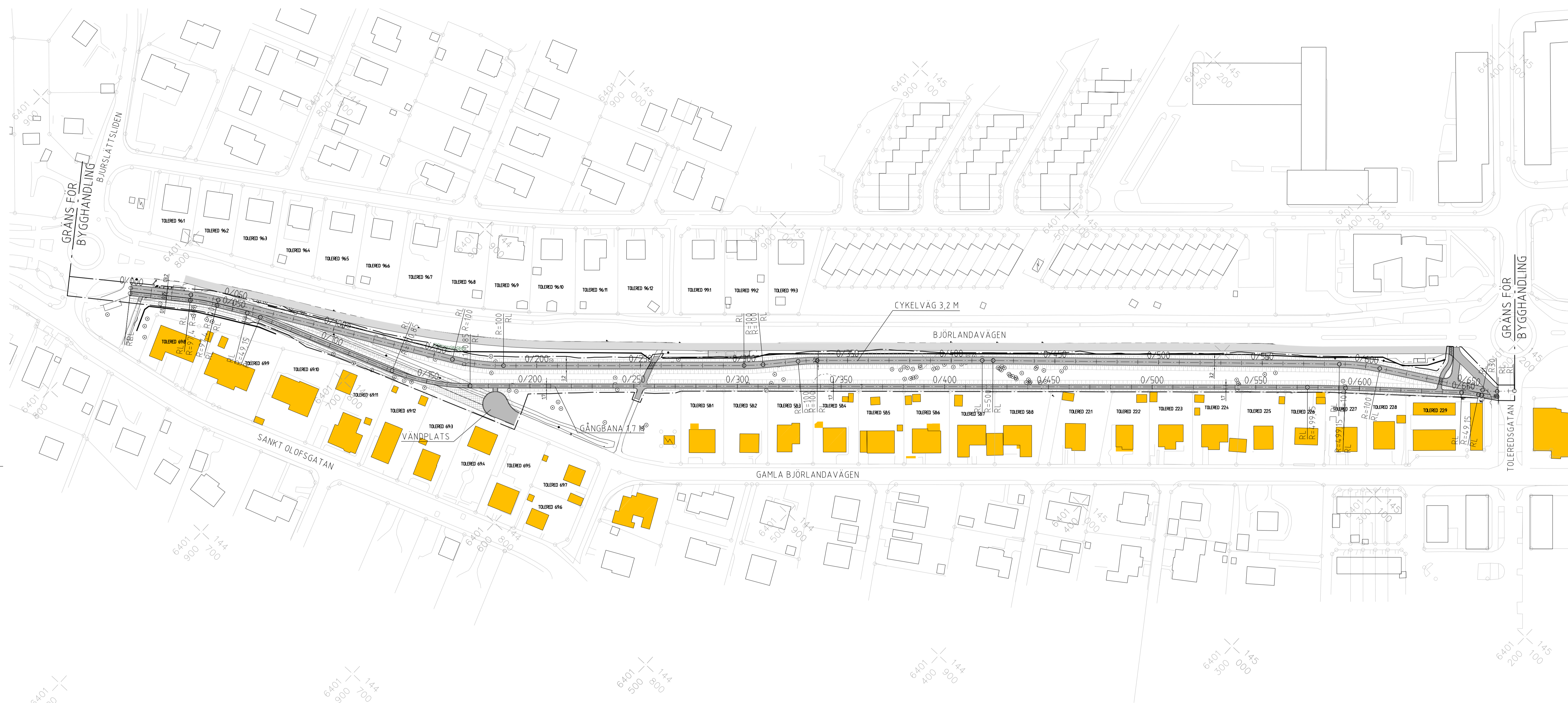
ÖVERSIKTSPLAN 1:1000
