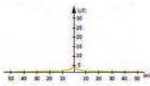
Figur 8.11.1. Magnetfältets styrka på olika avstånd från järnvägen när tåget är långt borta (mer än 2,5 kilometer bort). Strömstyrkan är 200 A och frekvensen 16,7 Hz.
