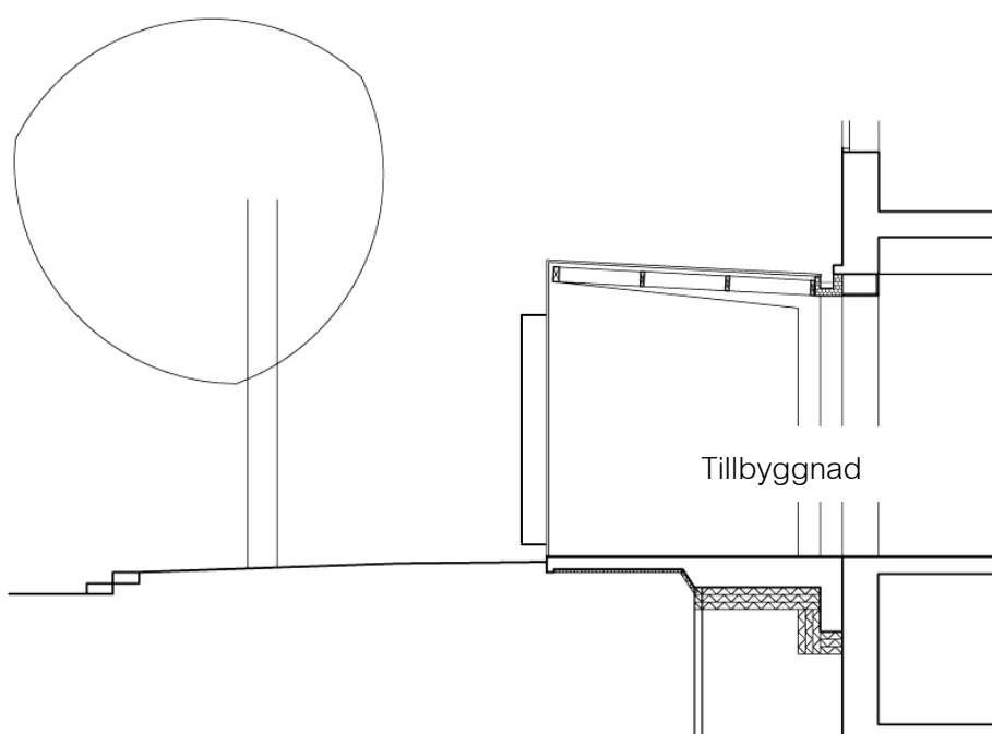
Principskiss konstruktion "balkong" 2014. Bestämmelse b2. Semrén & Månsson.
