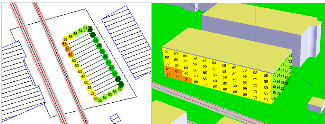
Bullerutredningen visar att den mest utsatta fasaden mot Theres Svenssons gata i huvudsak får värden <60 dBA. Det nordvästra hörnet av byggnaden kan om den högsta prognosen faller ut få värden marginellt överskridande 60 dBA.
