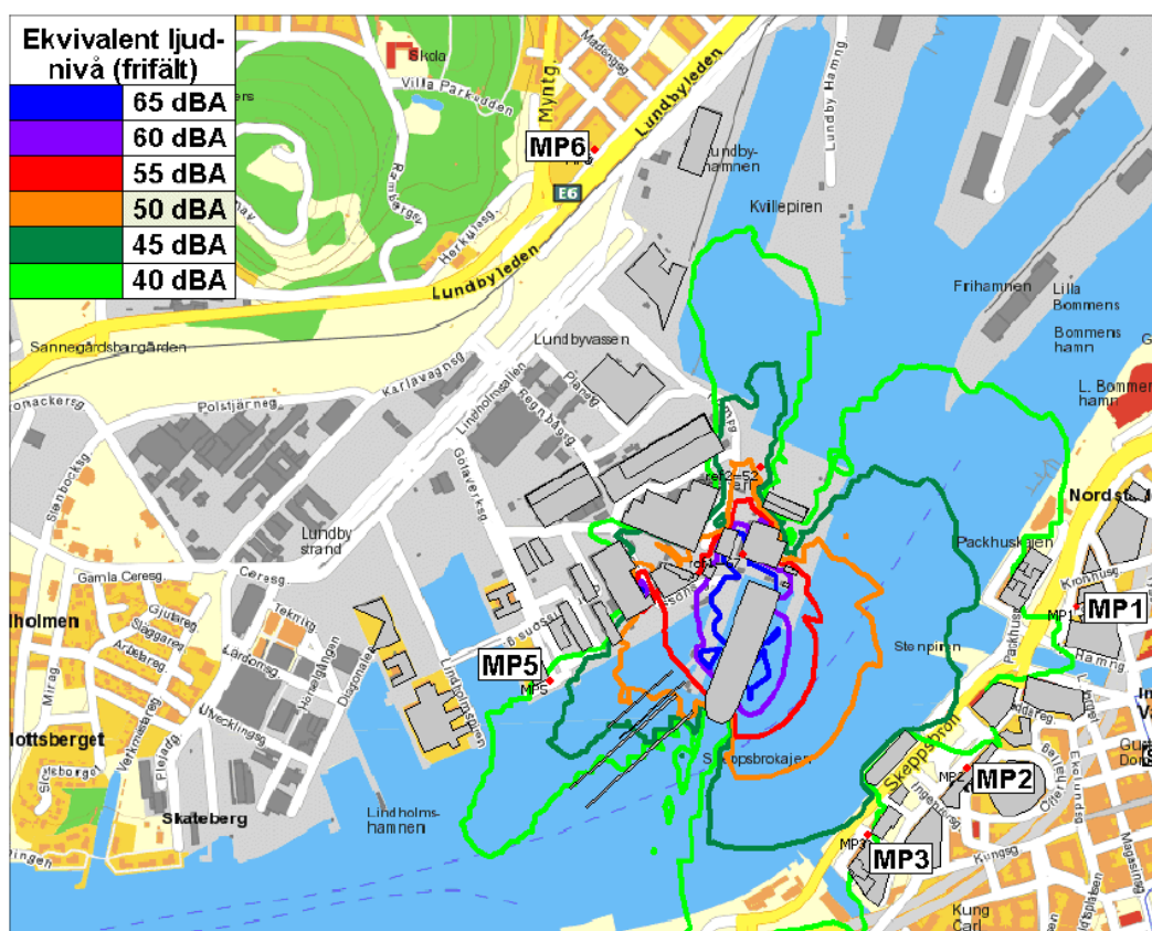
Ekvivalent ljudnivå från den tidigare varvsverksamheten vid Damen Ship Repair/Götaverken enligt ÅF:s bullerutredning "549269 Rapport A Externbullerkartläggning" daterad 2011-01-13.
