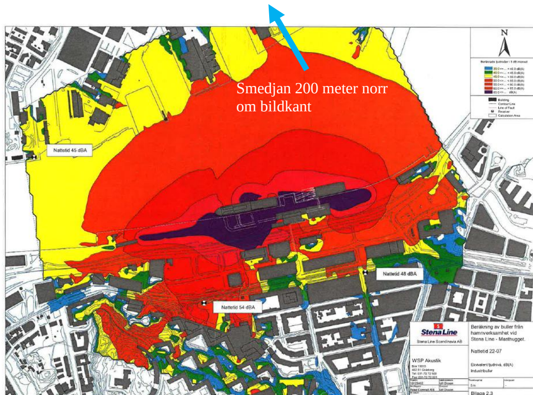
Bild från "Kartläggning av buller från fartyg och hamnverksamhet vid Masthuggsterminalen i Göteborg", WSP 2013-01-30. Bilden redovisar beräknade bullernivåer nattetid från Stena Lines terminal vid Masthuggskajen.
