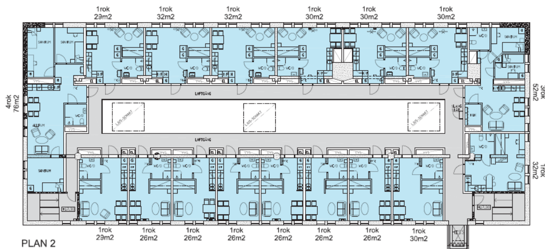
Planlösning efter ombyggnad till studentbostäder
