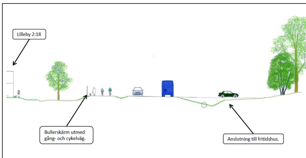
E.1:22 Illustration av sektionsutformning vid passage av bef bebyggelse, cirka km 1/800.
