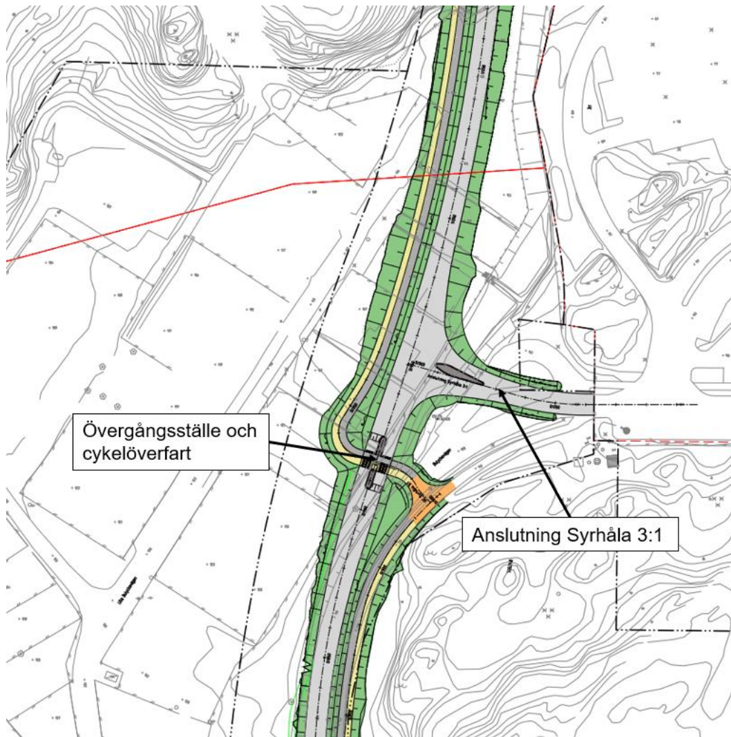
E.1:9 Planutformning 0/900-1/070.
