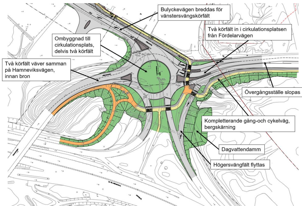
E.1:1 Syrhålamoet, utformningsförslag, delvis tvåfältig cirkulationsplats ersätter signalkorsning.
