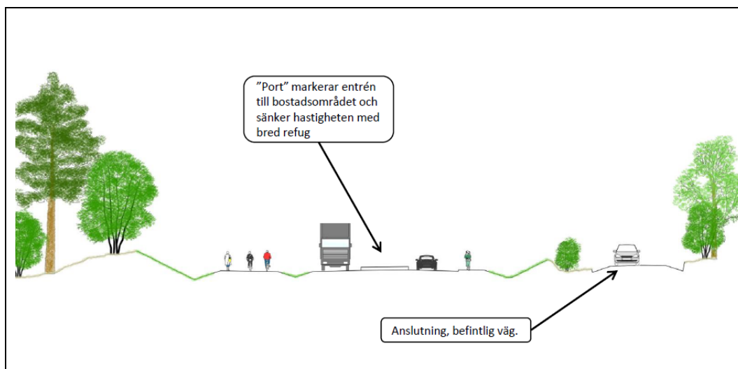
E.1:25 Illustration av sektionsutformning vid "porten" till Älvegårdsområdet, cirka km 2/100.
