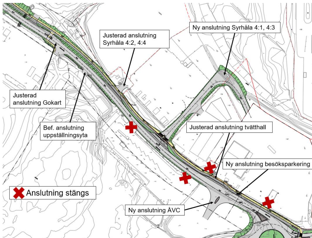
E.1:6 Stängning av anslutningar på sträckan 0/060-0/440.
