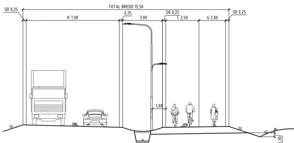
E.1:7 Typsektion 0/440-0/560
