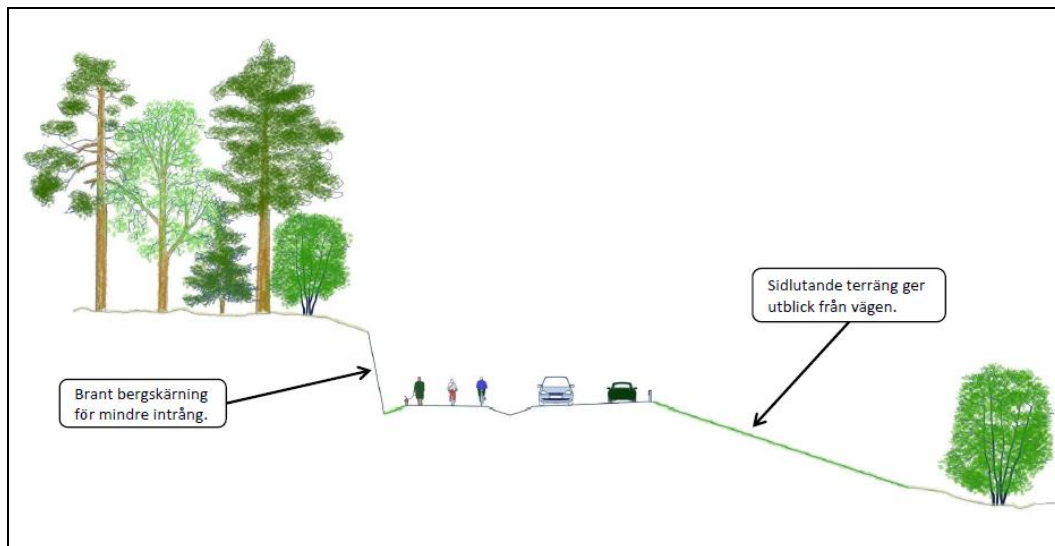
E.1:20 Illustration av sektionsutformning vid enkelsidig skärning, söder om kraftledningsgatan, cirka km 1/200.
