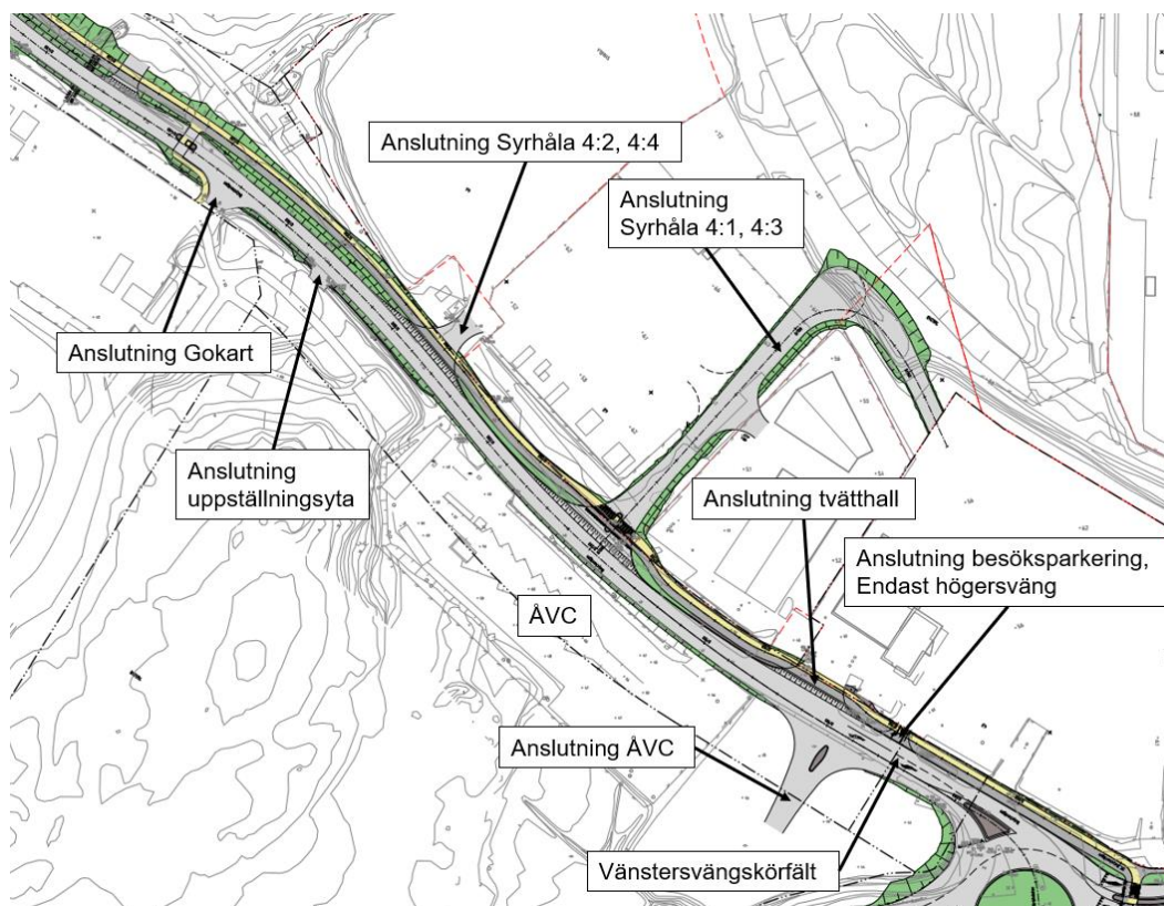
E.1:2 Planutformning 0/060-0/440.
