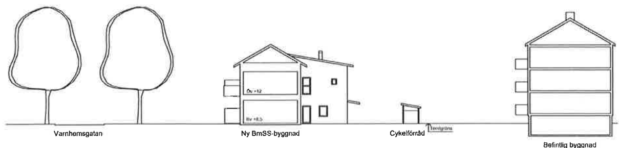
Figur 17. Sektion över föreslagen bebyggelse i relation till befintlig, Norconsult.
