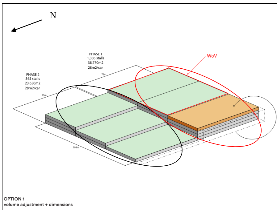
Figur 6 Preliminär skiss över World of Volvo ovanpå parkeringshuset. Röd ellips markerar del av parkeringshuset som är aktuell i denna detaljplan. Svart ellips markerar del av parkeringshuset som är aktuell i anslutande detaljplan (Inhouse Tech 2018).
