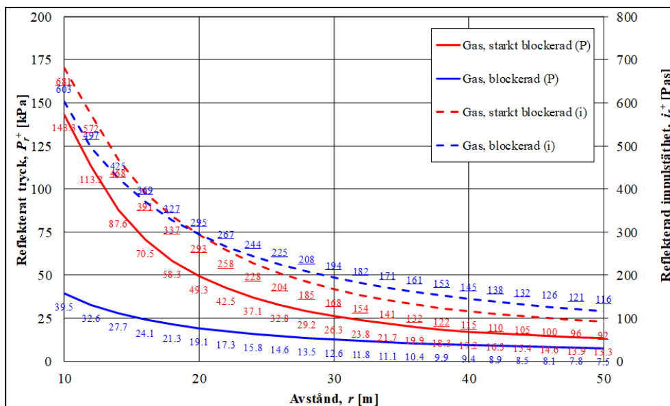
Figur 26. Lastvärden för explosionslast från blockerad samt starkt blockerad gasexplosion (Norconsult 2018).
