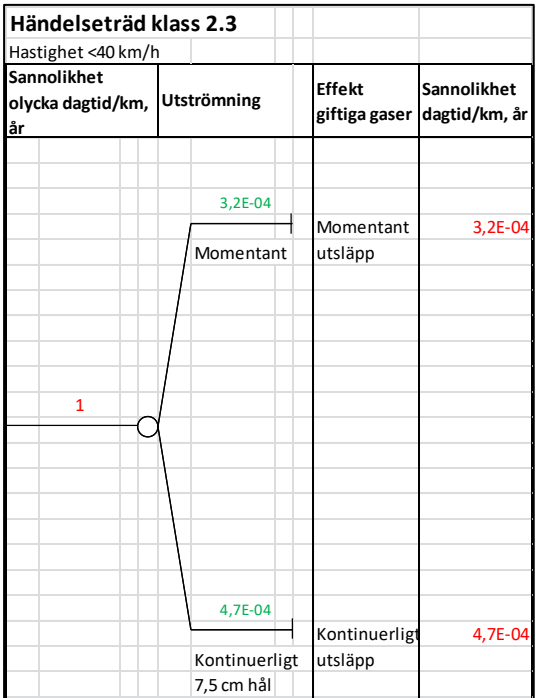
Figur 17. Händelseträd för olycka med giftiga gaser, tågastigheter under 40 km/h
