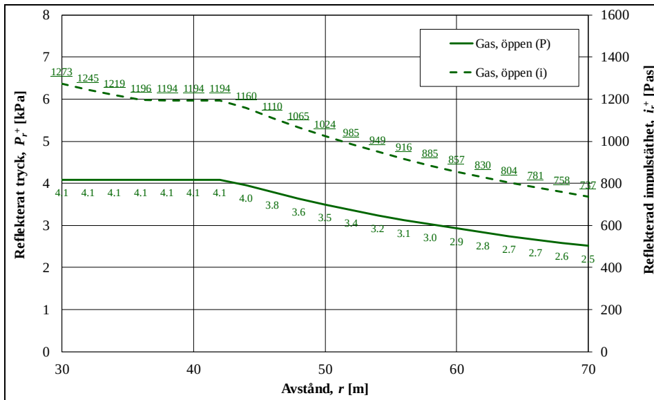
Figur 25. Lastvärden för explosionslast från en gasexplosion på en öppen yta (Norconsult 2018).
