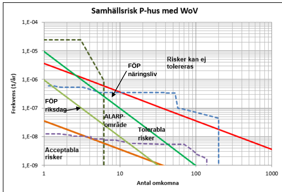
Figur 21. Samhällsrisk för P-huset och World of Volvo (WoV) från farligt gods på vägen (blå, streckat), järnvägen (lila, streckat), från urspärning (mörkgrön, streckat).
