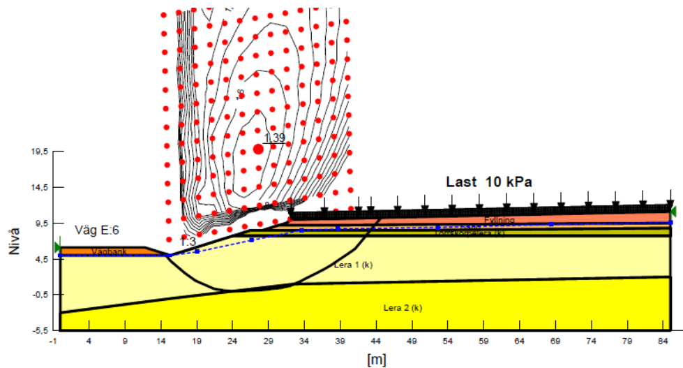
Figur 11 Sektion A, ökat lerdjup (kombinerad analys)
