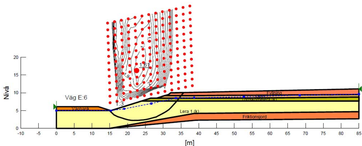
Figur 9 Sektion A, befintliga förhållanden (kombinerad analys).
