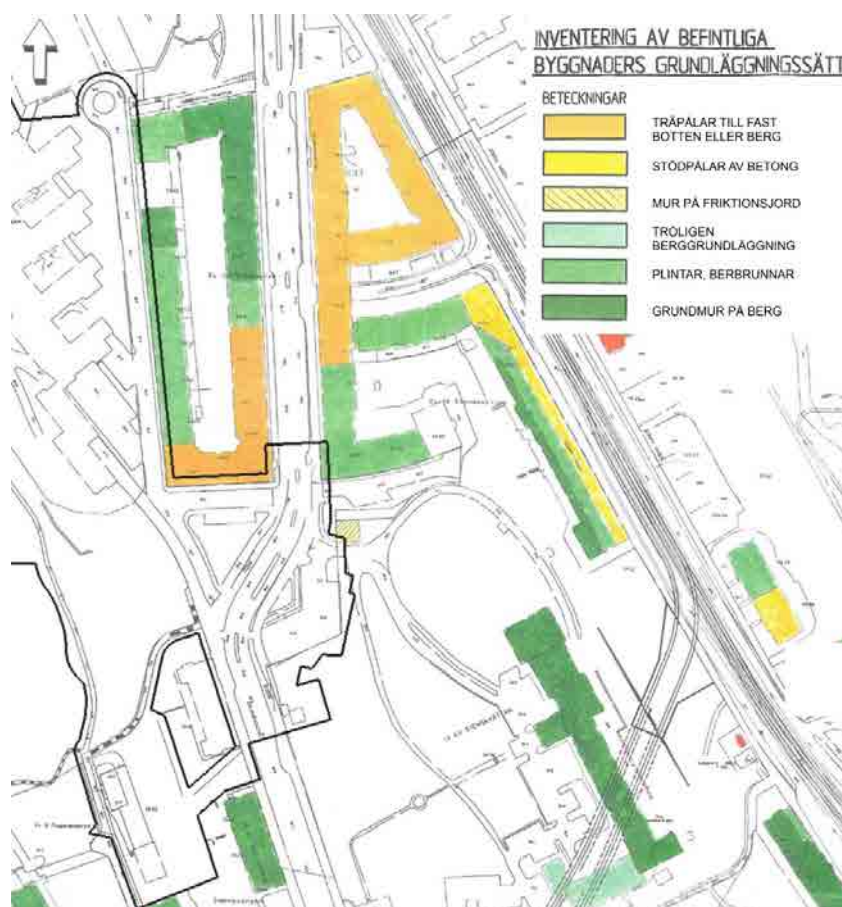
Figur 5.6. Inventering av befintliga byggnaders grundläggningssätt vid byggnation av Kringen. Modifierad bild från GF Konsult, Tekniskt PM angående grundvattensänkning och sättningar. 1998-12-14
