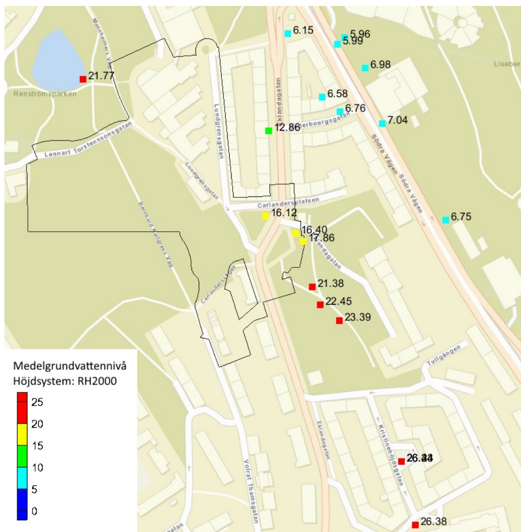
Figur 5.3. Medelvärde av grundvattennivåer i jord, undre magasin.
