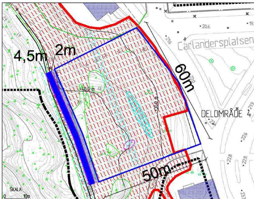
Figur 4.1. Maximalt utnyttjande av området för eventuell ny byggnad vid Carl- andersplatsen (tjockt blått streck). Längs Bernhard Karlgrens Gångväg (heldragna vita streck) visar blå skraffering en linje 2 m respektive 4,5 m utanför maximal byggbar area. För övriga symboler hänvisas till teckenförklaring i Bilaga 2.
