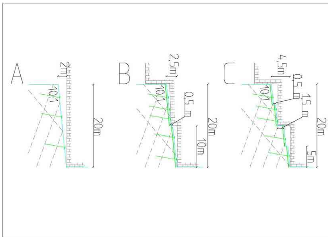
Figur 4.2. Förslagsskiss för uttag och förstärkning. Blått: teoretisk släntkontur. Grönt: förstärkning. Streckat grått: sprickor. A: uttag i en enda 20 m hög pall med permanentförstärkning. Teoretiskt släntkrön 2 m utanför byggnadens vägg. Endast grundläggning på schaktbotten. B: Uttag i två pallar med 0,5 m bred hylla för att kunna utföra förförstärkning (10 m långa bultar parallella med teoretisk släntkontur). Teoretiskt släntkrön 2,5 m utanför byggnadens vägg. Grundläggning även på teoretisk släntkrön. C: Uttag i fyra pallar med en 1,5 m bred berghylla. Teoretiskt släntkrön 4,5 m utanför byggnadens vägg. Grundläggning även på teoretisk släntkrön.
