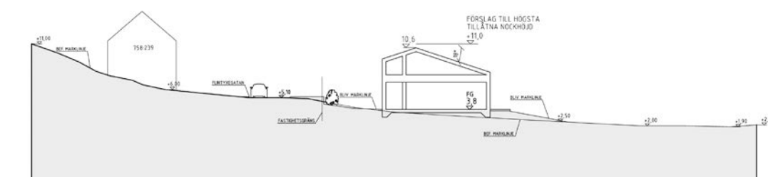
SEKTION C-C
