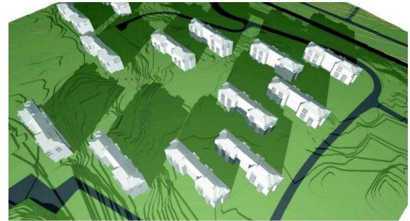
Skuggorna på vårdagjämningen klockan 17:00 före och efter påbyggnad, sett från sydväst.
