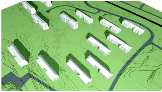
Skuggorna på vårdagjämningen klockan 15:00 före och efter påbyggnad, sett från sydväst.
