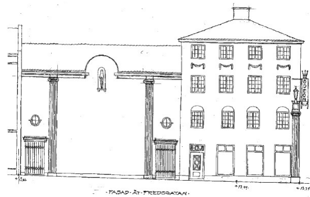
Biograf Odéon, ritningar från 1917 då tre äldre byggnader byggdes om och till för att fungera som biograf. Källa:
