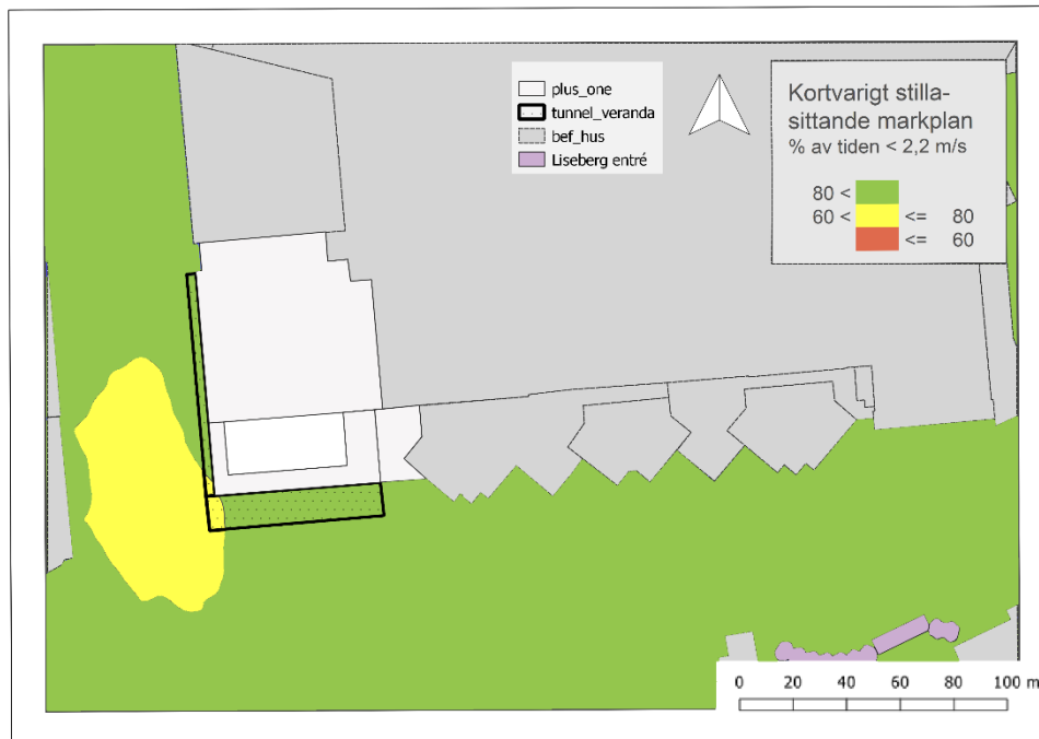
Figur 8 Vindkomfort för kortvarigt stillasittande på verandan i markplan (prickigt område). Resultatet visar antal timmar (i %) under ett år där vinden är <2,2 m/s. Färgerna motsvarar klassifikationen i Tabell 4.
