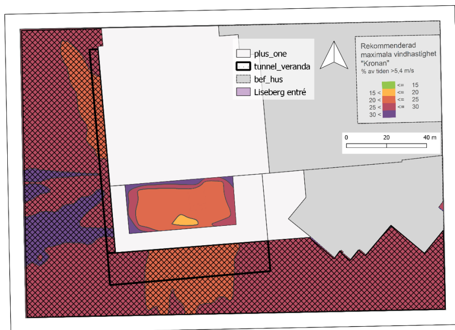
Figur 13 Rekommenderad maximal vindhastighet enligt Oke m.fl. (2017) på takterrassen Kronan. Resultatet visar antalet timmar (i %) under ett år där vinden >5,4 m/s på en höjd 131 meter över markplan.
