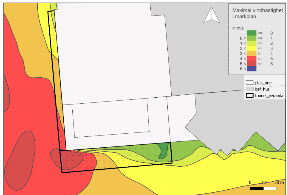
Figur A 3 Maximal vindhastighet i markplan, resultatet visas i m/s.
