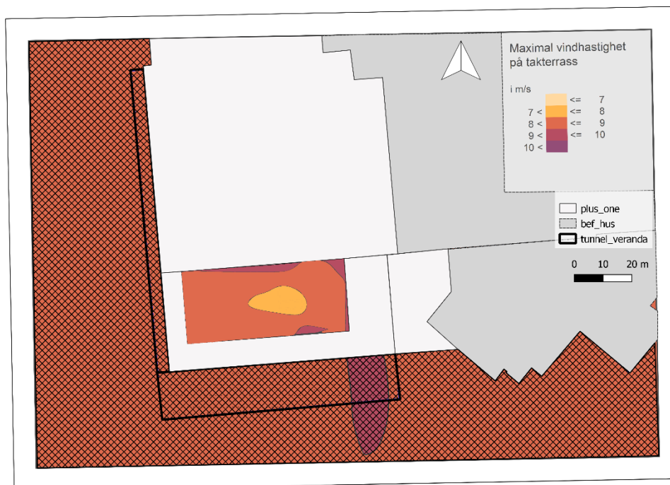
Figur 14 Maximal vindhastighet under ett typår, på takterrassen Kronan. Resultatet visas i m/s på en höjd 131 meter över markplan (prickigt område).
