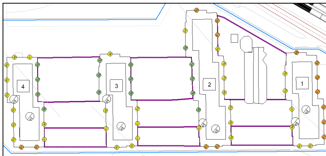
Figur från bullerutredningen. Orange punkter markerad de delar av fasaden där särskilda åtgärder krävs. Utan åtgärder ligger de ekvivalenta bullernivåerna på mellan 61-63 dBA. Med hjälp av avskärmning och rumslig ljuddämpning kan ljudnivån sänkas med 1-8 dBA för de mest bullerutsatta bostäderna.
