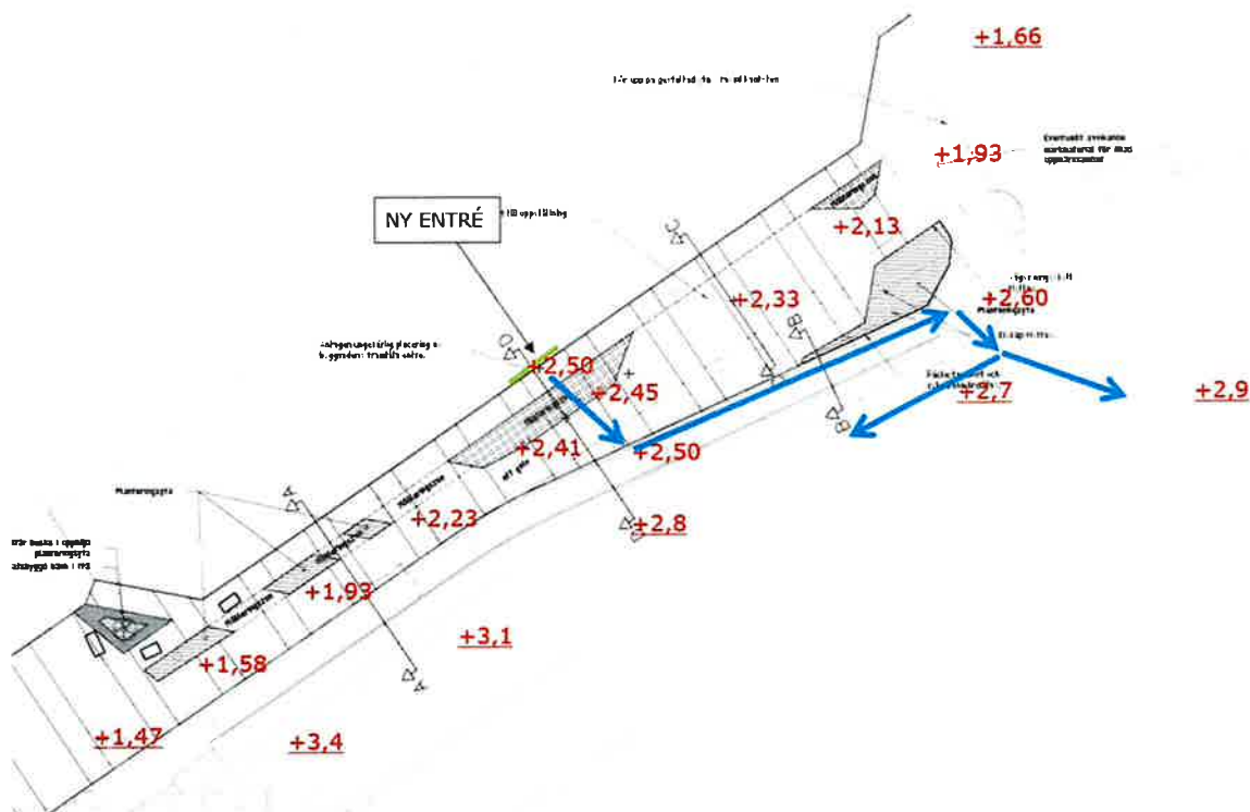
Figur 41: visar ny höjdsättning av Kilsgatan i östvästlig sträckning (Ramboll 2023). Befintliga höjder är understruckna, nya höjder inte. Grönt streck markerar ny entré. Blå pilar visar utrymningsväg från ny entré vid en högvattensituation på +2,3.
