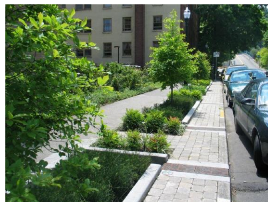
Seriekopplade raingardens
