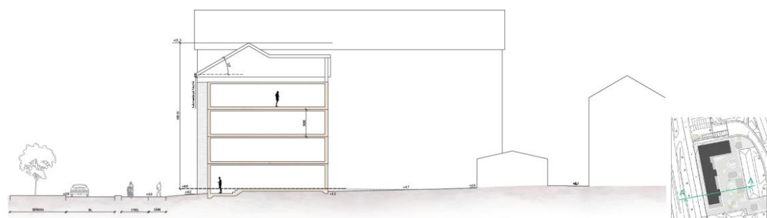
Sektion A-A.
