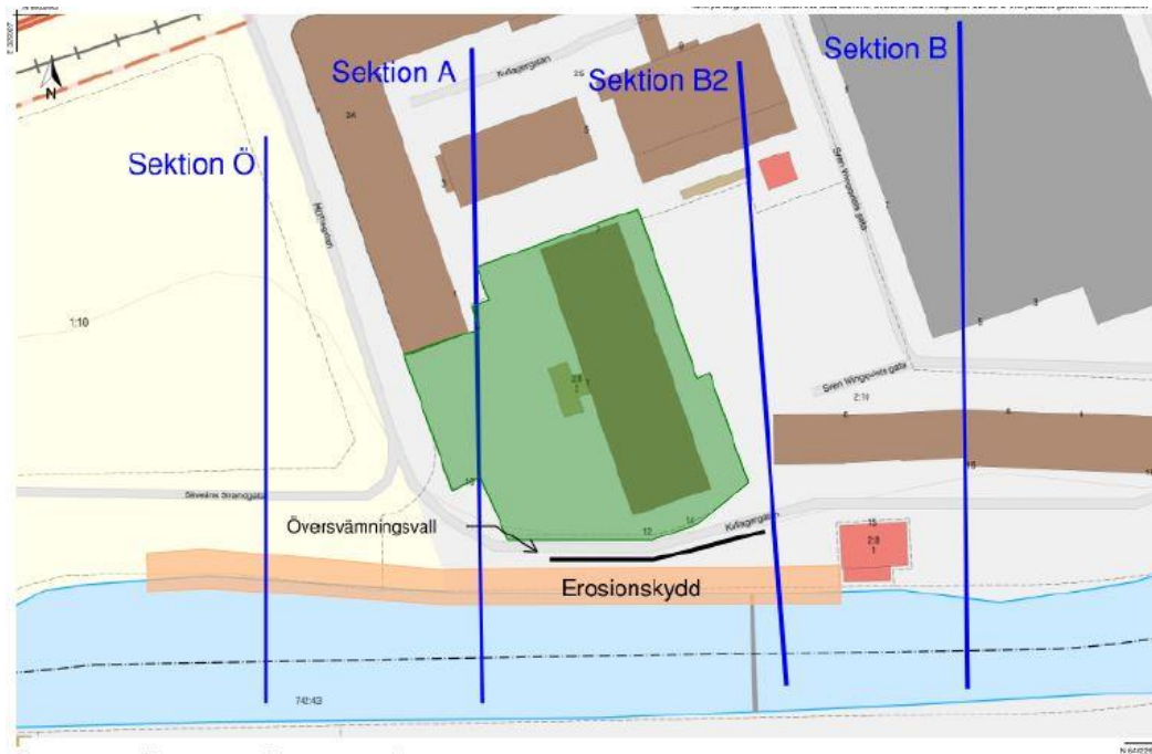
Plan som visar sträckan längs Säveån där befintligt erosionsskydd behöver förbättras. WSP, år 2021
