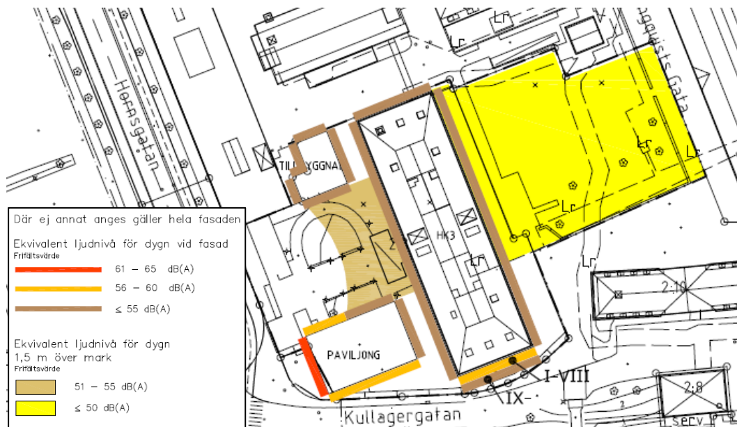
Bullersituationen, prognos år 2040, ÅKERLÖF HALLIN AKUSTIKKONSULT år 2021
