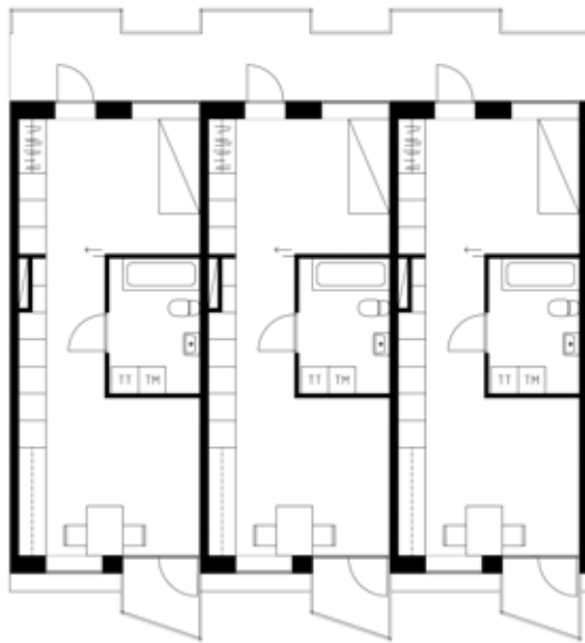
Typlägenheter norra kvarteret White arkitekter
