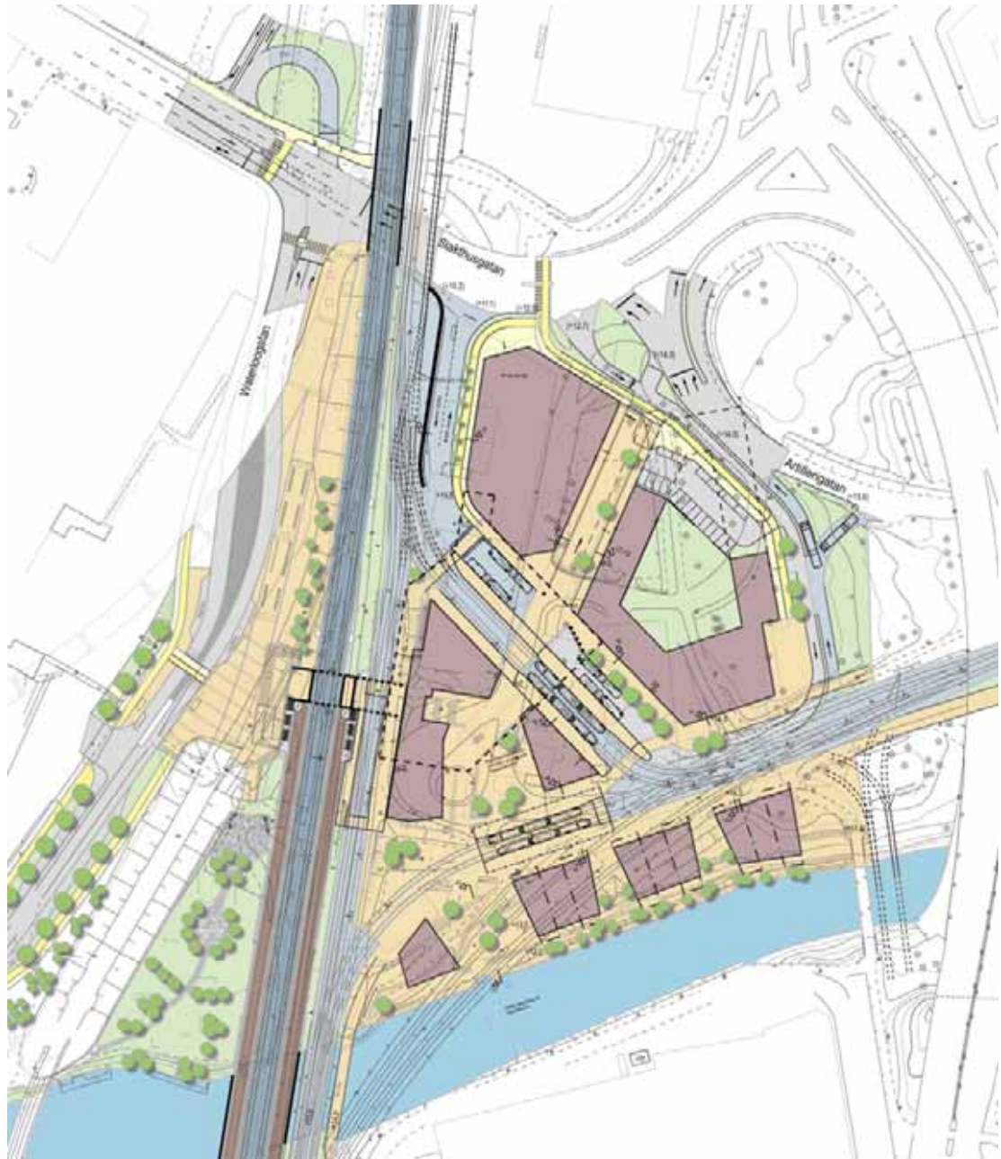
Trafik- och gestaltningsförslaget för utformning av kollektivtrafikytor, gator och platser i etapp 1. Justeringar har skett inför utställning - se plankarta samt särskild illustrationskarta av mark och trafik. Trafik- och gestaltningsförslaget redovisar en alternativ utbyggnad med en minskad byggnation utmed Artillerigatan m.a.a. byggnation av vägtunneln.
