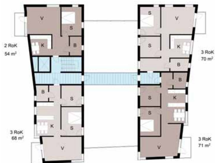
Typlägenheter kajhusen
