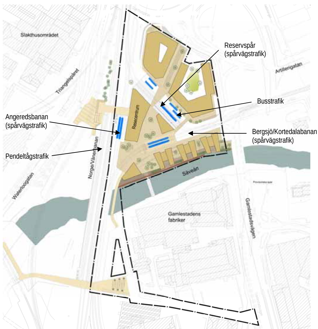
Illustration av planförslaget med den nya lösningen för knutpunkten. Illustration: White arkitekter
