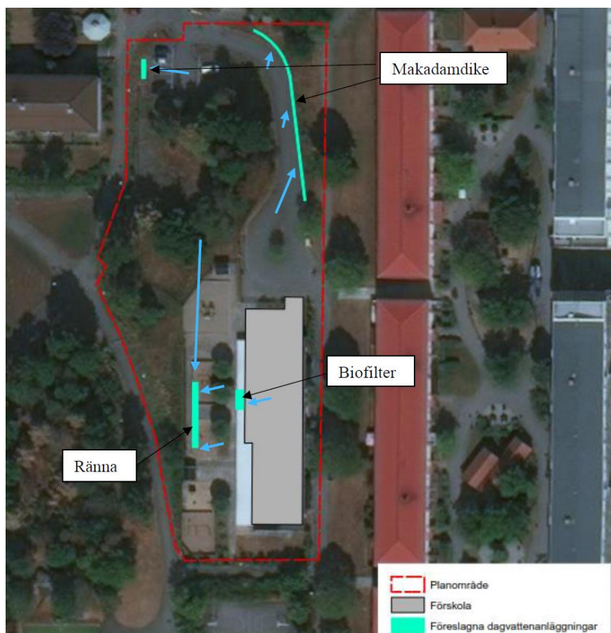
Föreslagna dagvattenanläggningar vid Saffransgatans förskola. Blå pilar visar ungefärlig avrinning.
