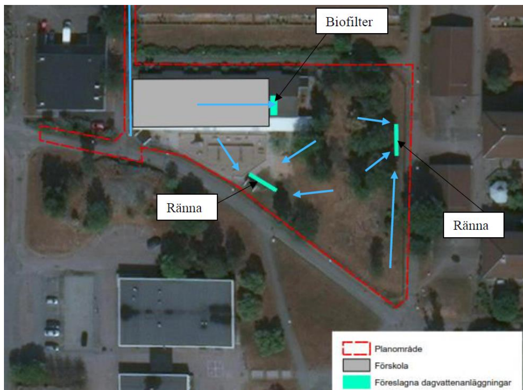
Principlösning för dagvattenhantering vid Timjansgatan. Blå pilar visar ungefärlig avrinning.
