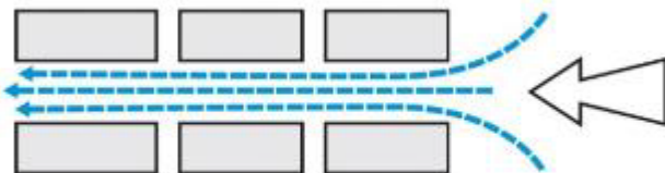
Figur 34 -vindtunneleffekt kan oppstå dersom gatebredden er mindre enn 0,5 \times bebyggelsens høyde, og dersom gaten ligger parallelt med framherskende vindretning. Denne effekten vil oppstå i gater som er lengre enn 100-125 meter.
