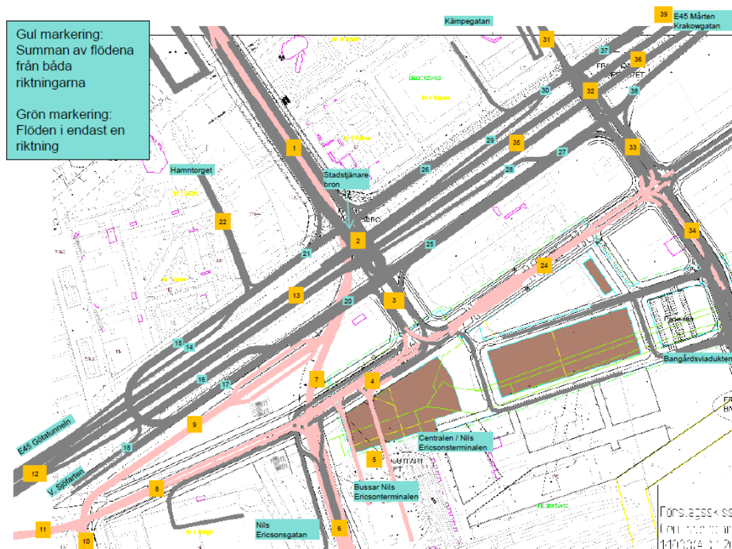
Figur 2. Mätpunkter trafik.
