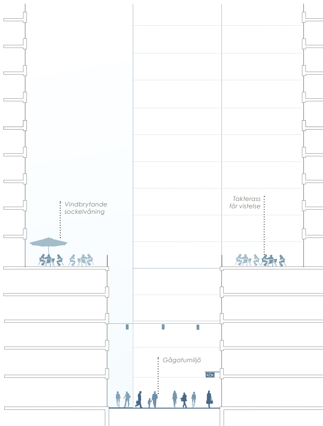
Principsektion genom stråket
