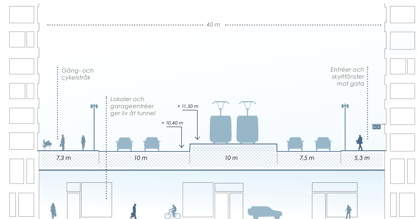
Principsektion genom Stadstjänaregatan i korsningen med Gullbergs strandgata. Brorampens höjd i detta läge är ca 10 meter och spårvagnsrampen är nästan i nivå med resten av rampen. Brorampens ovansida sträcker sig från fasad till fasad och Gullbergs Strandgata passerar under Stadstjänaregatan.
