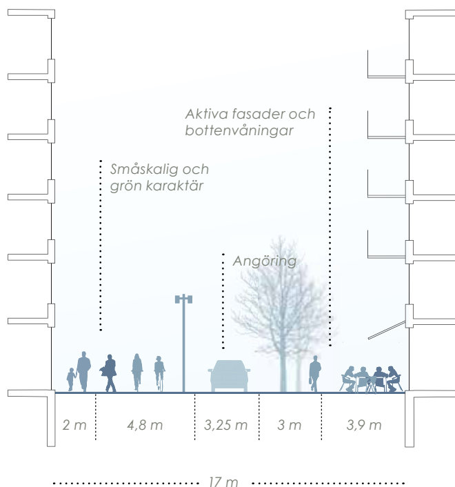
Principsektion genom stråket i Lilla Bommen-området
