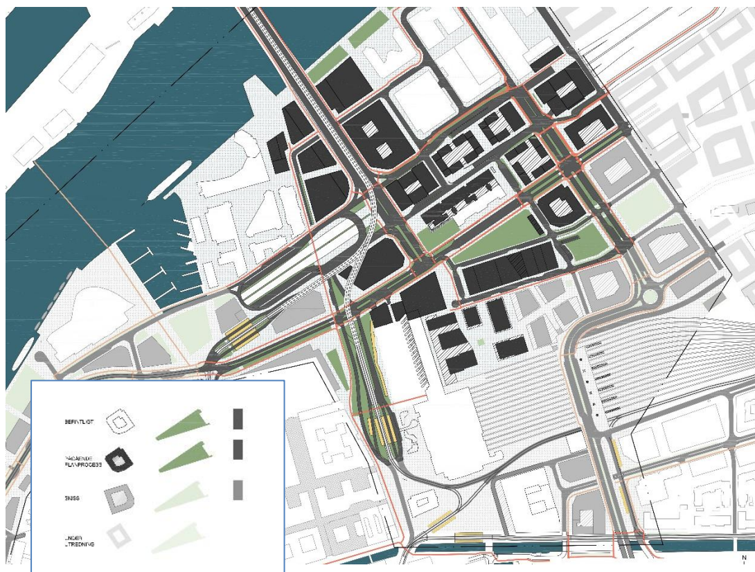
Planstruktur för Centralenområdet 2040. Biltrafik och huvudgatusystem i grått, huvudcykelstråk i orange. Bild stadsbyggnadskontoret
