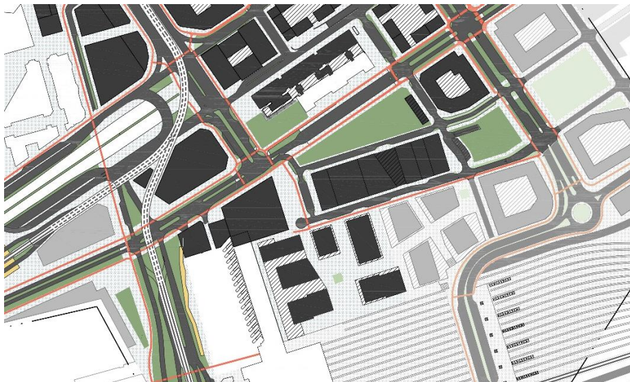
Planstruktur för Centralenområdet 2040. Biltrafik och huvudgatusystem i grått, huvudcykelstråk i orange. Bild stadsbyggnadskontoret
