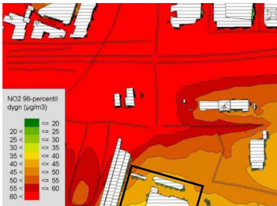
Luftkvalitetsberäkning med CFD-mo- dell. Planområde markerat. Bild COWI.
