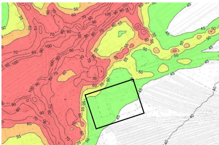
Luftkvalitetsberäkning med gaussisk model. Planområde markerat. Bild SWECO
