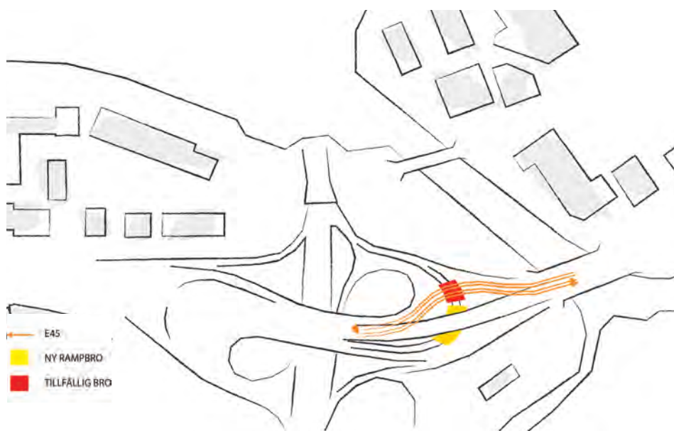
Figur 3.19. Omledning av trafik på E45 vid nybyggnation av rampbro i Gullbergsmotet.
