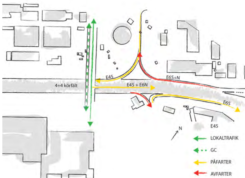
Figur 3.15. Illustrationsplan för Falutorget och trafiklösning med en vänsterpåfart från lokalbron.
