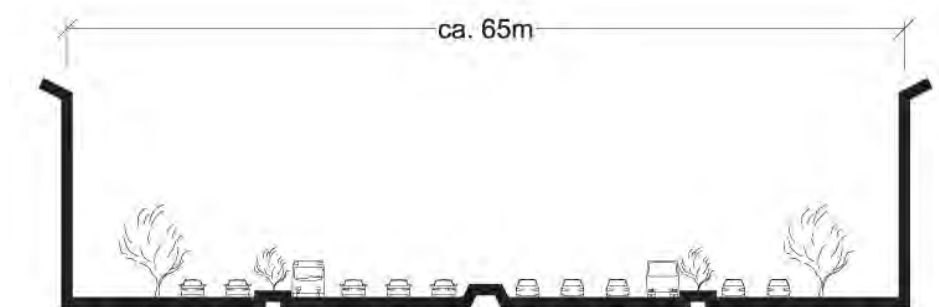
Figur 3.14. Sektion som illustrerar kommunens förslag om stadsgata.
