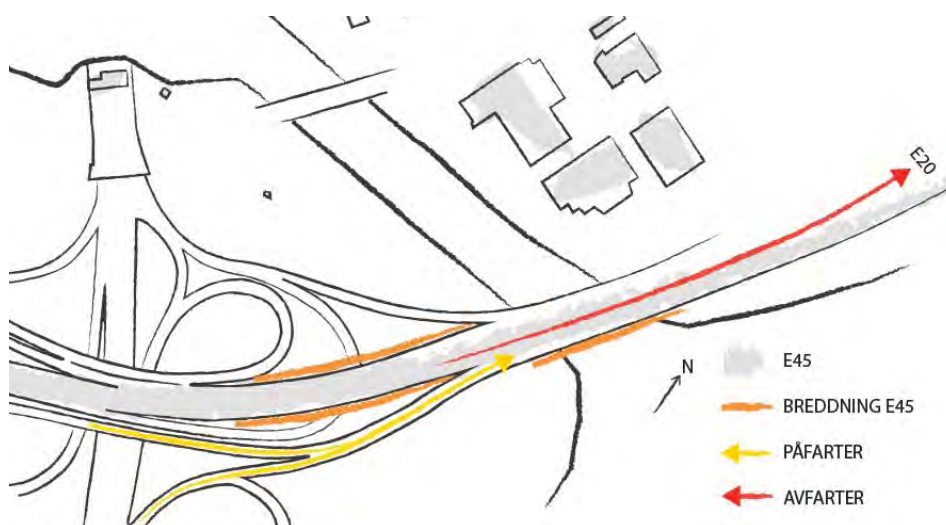
Figur 3.16. Illustrationsplan av trafiklösning vid Sävån med ett extra körfält över Sävån.
