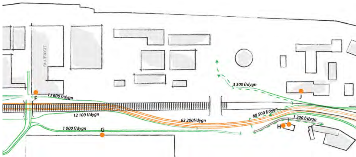
Figur 4.5. Tillfälliga vägar etapp 2.
