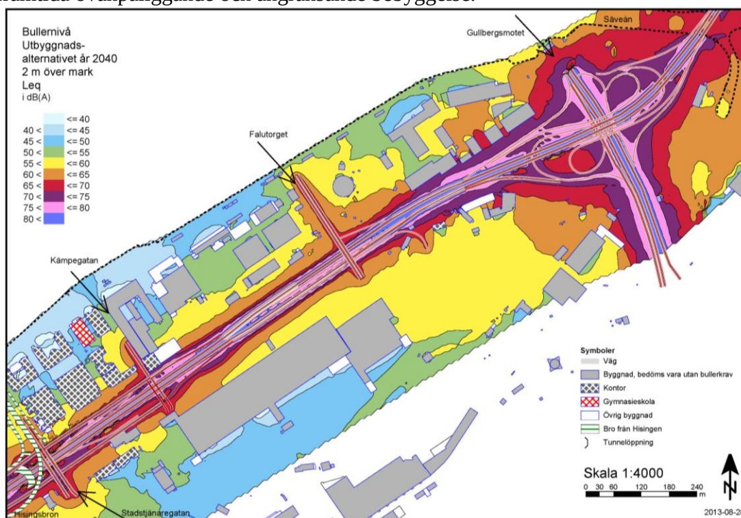
Figur 26, Kartan visar ekvivalenta ljudnivåer, 2 meter över mark, framtagna efter trafikscenariot år 2040 (av Tyréns för Trafikverket).
