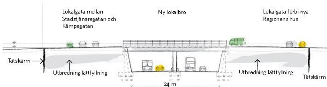
Figur 18, principsektion över ny lokalbro vid Kämpegatan med 2+2 körfält (av Tyréns AB för Trafikverket).
