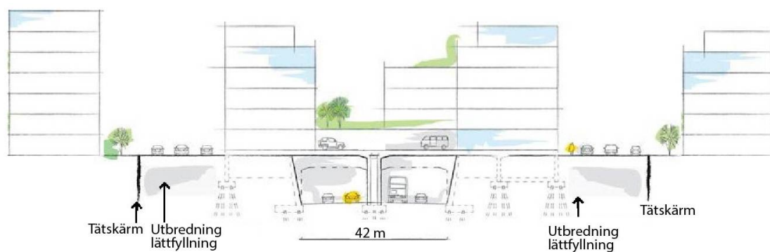
Figur 14, principsektionen illustrerar ett möjligt sätt att i framtiden kunna bygga på nedsänkningen med byggnader (av Tyréns AB för Trafikverket).
