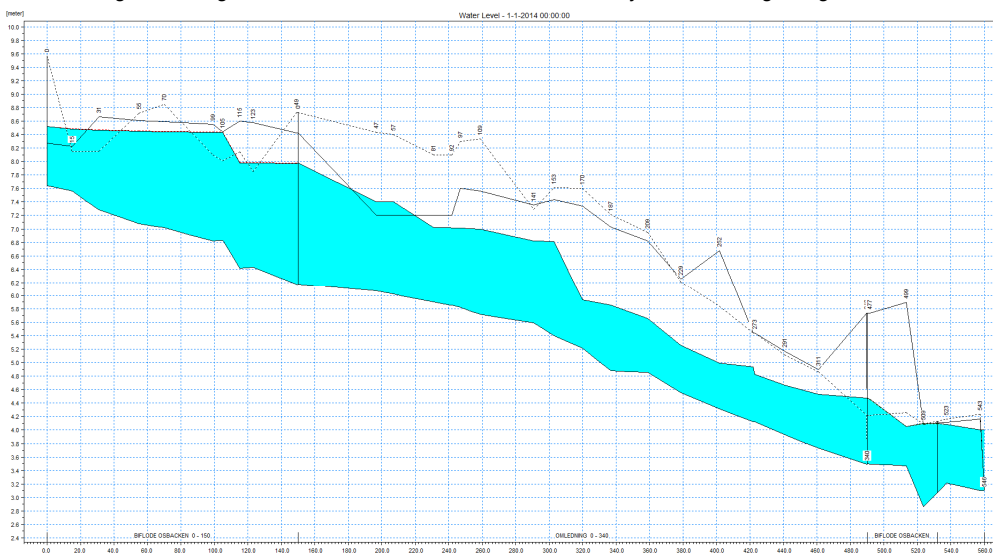
Figur 13. HHQ 50 för situation med omledning av bäck. Det blå visar vattennivån från botten till ytan. Linjerna med siffror visar slänkrönet för respektive tvärsektion.
