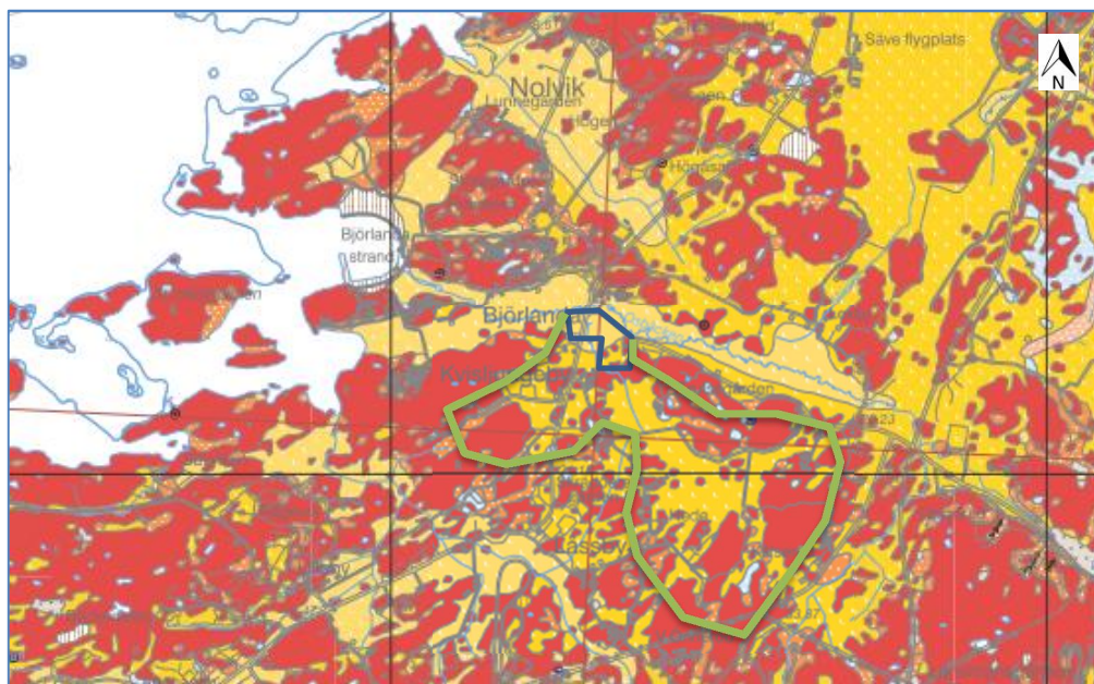
Figur 2. Utsnitt ur SGUs jordartskarta. Rött illustrerar berg i dagen, mörkgult-glacial lera, ljusare gul ton-postglacial lera och orange med vita prickar olika fraktioner av postglacial sand och svallsediment. Blå linje visar planområdet och grön linje visar ungefärlig avgränsning av avrinningsområdet för bäcken som rinner genom och avvattnar planområdet idag.
