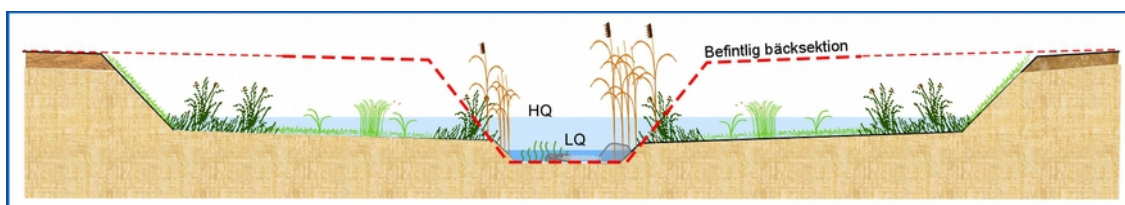
Figur 3. Bäcksektion av tvåstegstyp med översvämningsytor och viss flödesutjämnande effekt.
