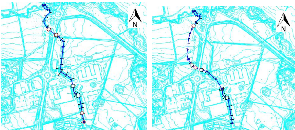
Figur 9. Modelluppställning för befintlig situation till vänster och omgrävningsalternativ till höger.
