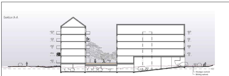
Sektion A-A
