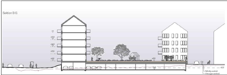
Sektion B-B
