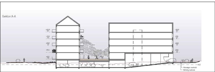
Sektion A-A
