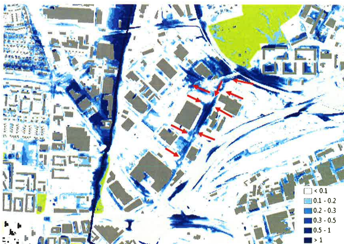
Beräknad översvänningsutbredning och vattendjup (m) för dagens situation. Röda pilar indikerar flödesriktning vid Backavägen.
