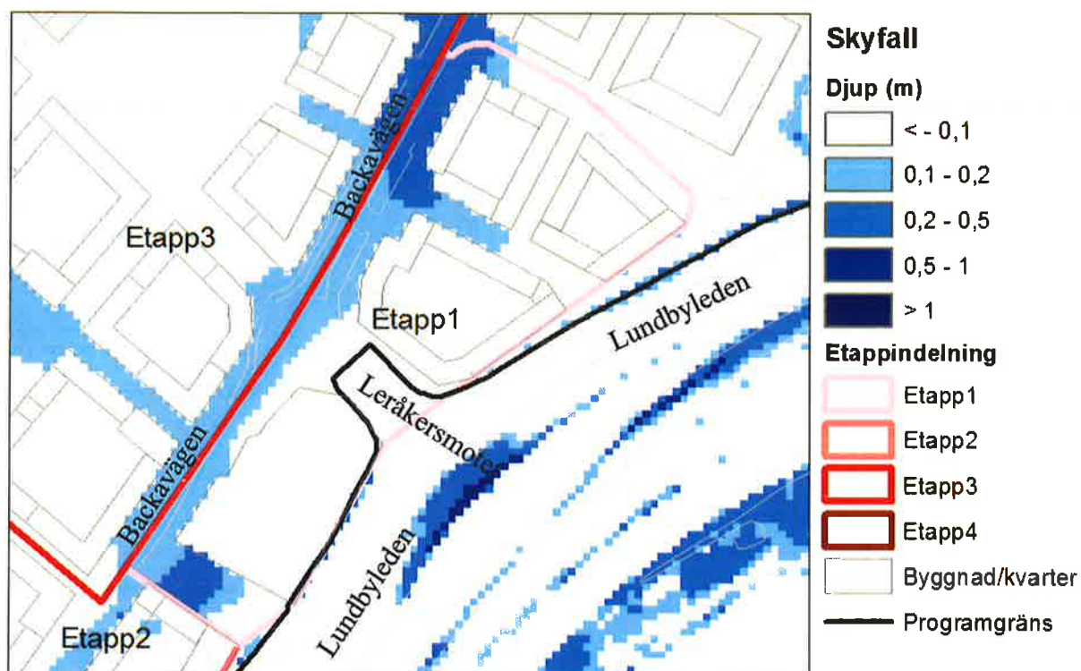
Figur 1. Översvänningsutbredning i etapp 1 vid framtida 100-årsregn (år 2100).
