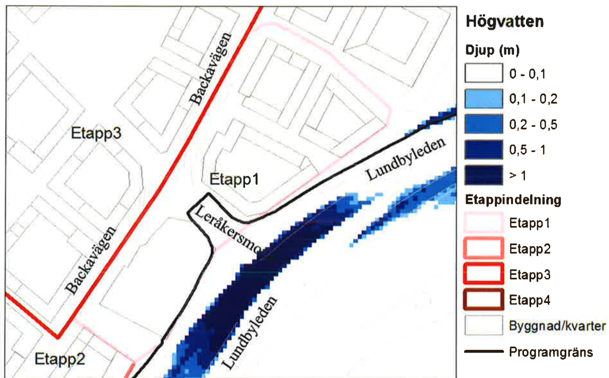
Figur 2. Utvärdering av högvattenrisk för etapp 1. Figur visar djup vid nivån +2,27 m i Göta älv (högvattennivå år 2070).
