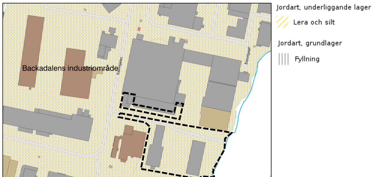
Figur 7. Jordartskarta 1:25 000 - 1:100 000 (SGU, 2021).
