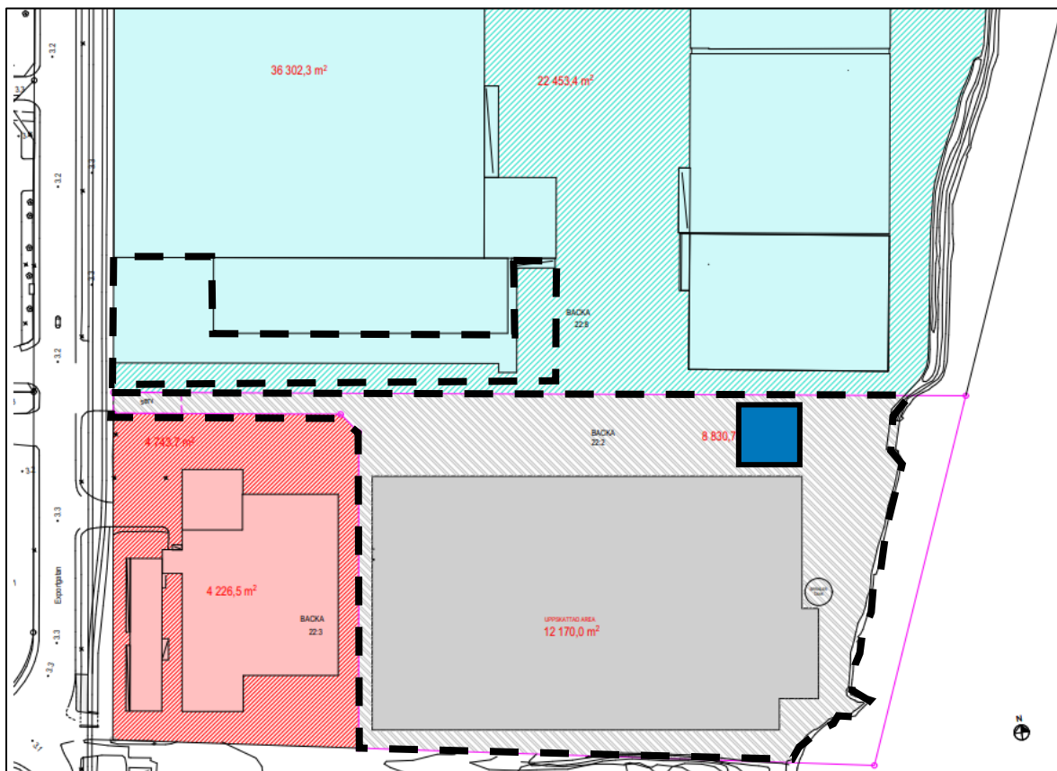
Figur 1. Föreslagen principiösning för dagvattenhantering. Blåmarkerat område visar föreslagen placering av magasin.
