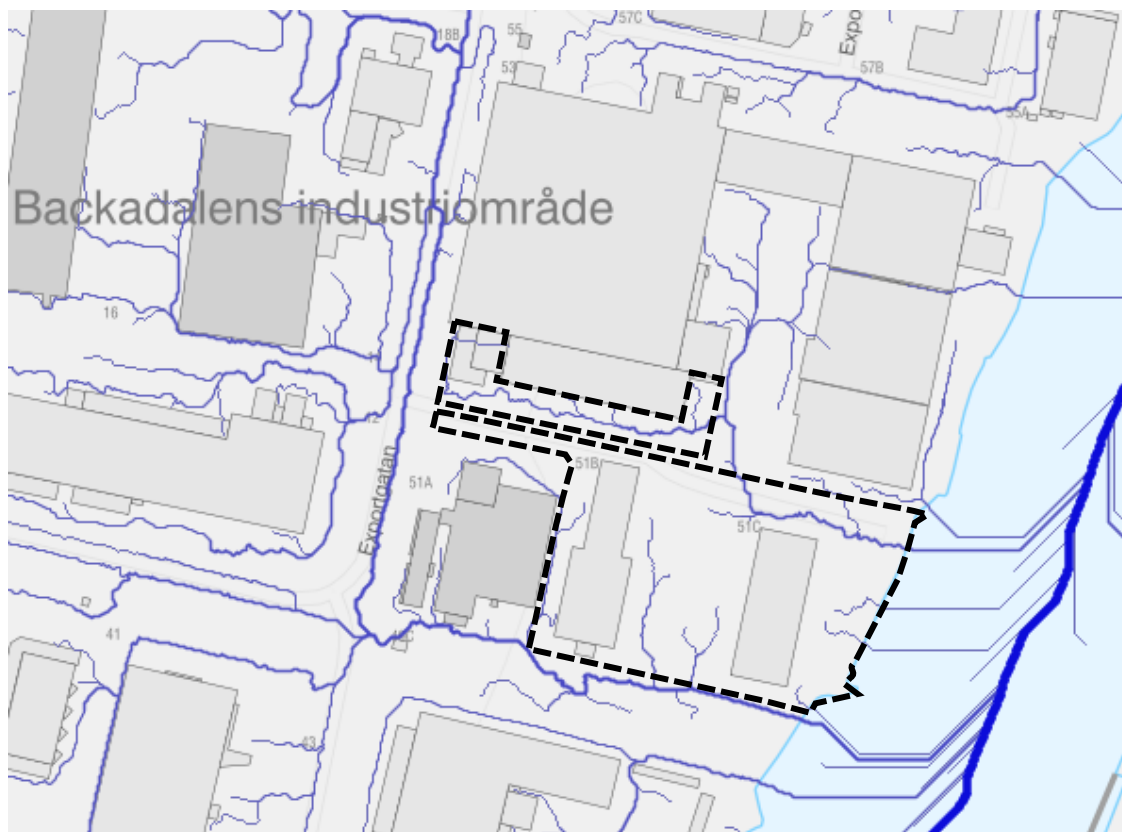
Figur 6. Översiktlig avrinning inom utredningsområdet (Scalgo Live, 2021).
