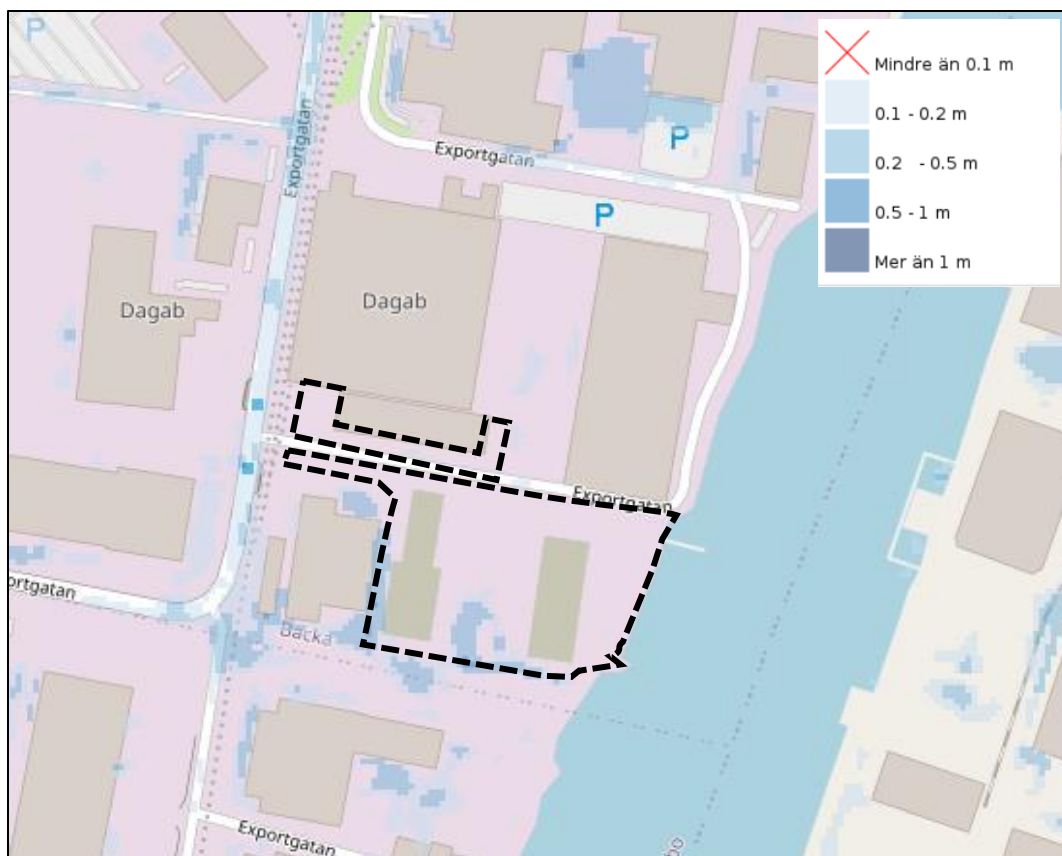
Figur 13. Blå områden visar vattendjup vid skyfall i området. Utredningsområdet är markerat med svart streckad linje (Stadsbyggnadskontoret, u.d.).
