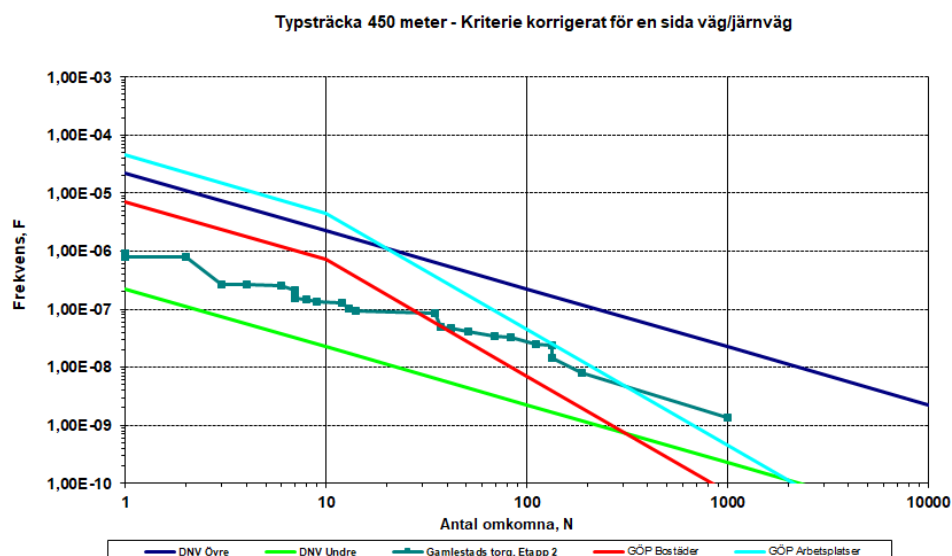
Figur 14. Samhällsrisk för studerat planområde och befintlig bebyggelse inom utredningsområdet efter etablering i enlighet med beskrivningar i kapitel 3, med hänsyn till riskreducerande åtgärder på ny bebyggelse.
