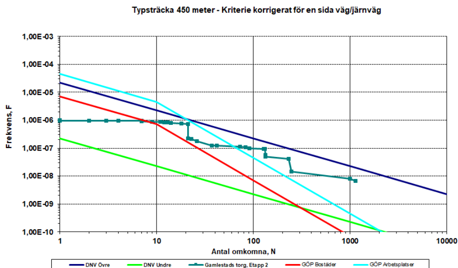
Figur 13. Samhällsrisk för studerat planområde och befintlig bebyggelse inom utredningsområdet efter etablering i enlighet med beskrivningar i kapitel 3, utan hänsyn till riskreducerande åtgärder på ny bebyggelse.
