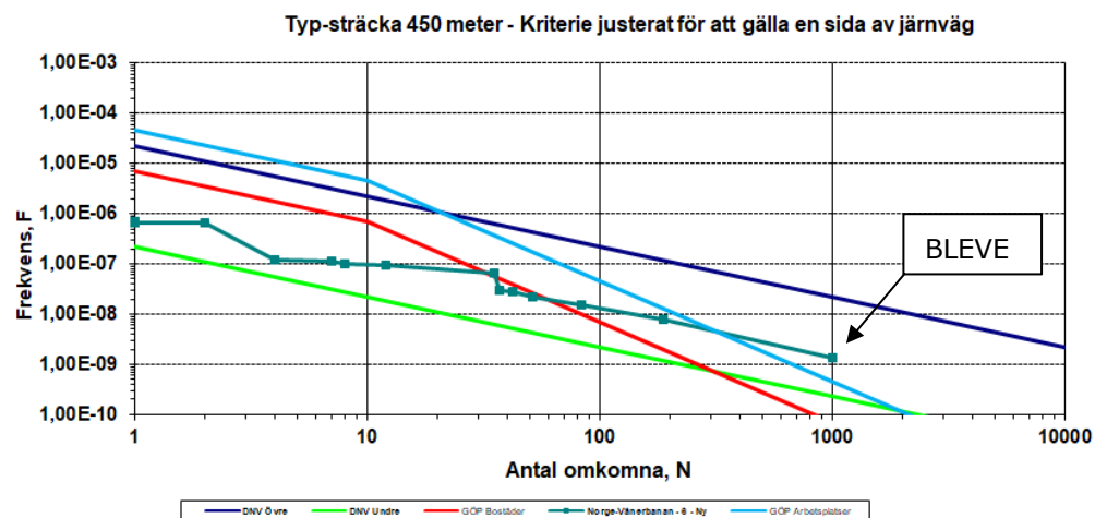
Figur 15. Samhällsriskerna för enbart de verksamheter som planeras inom utredningsområdet, med hänsyn till riskreducerande åtgärder.
