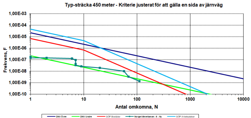
Figur C.1. Samhällsrisk för enbart bostäder när ventilation placeras högt och vänd från järnvägen.
