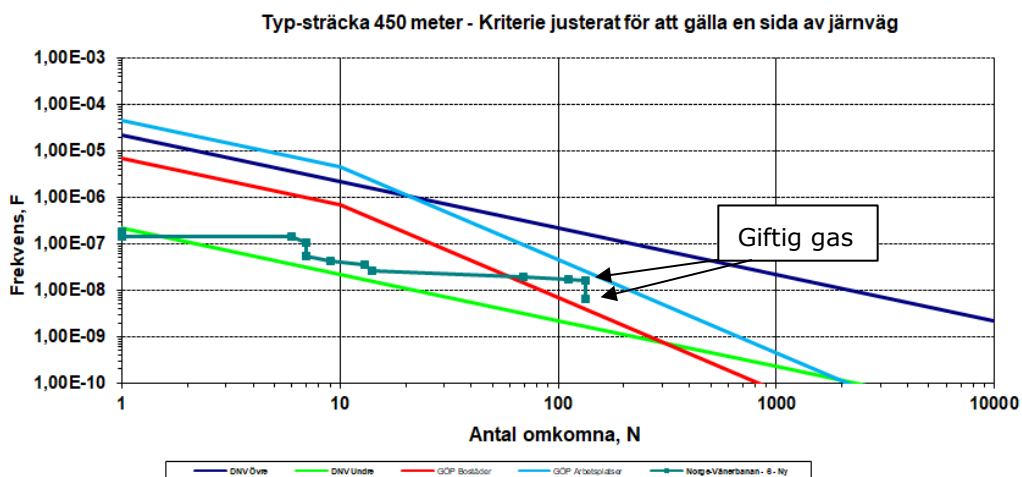
Figur 16. Samhällsrisknivån för enbart de bostäder som planeras inom utredningsområdet. Inga rekommenderade skyddsåtgärder har kvantifierats för dessa bostäder.
