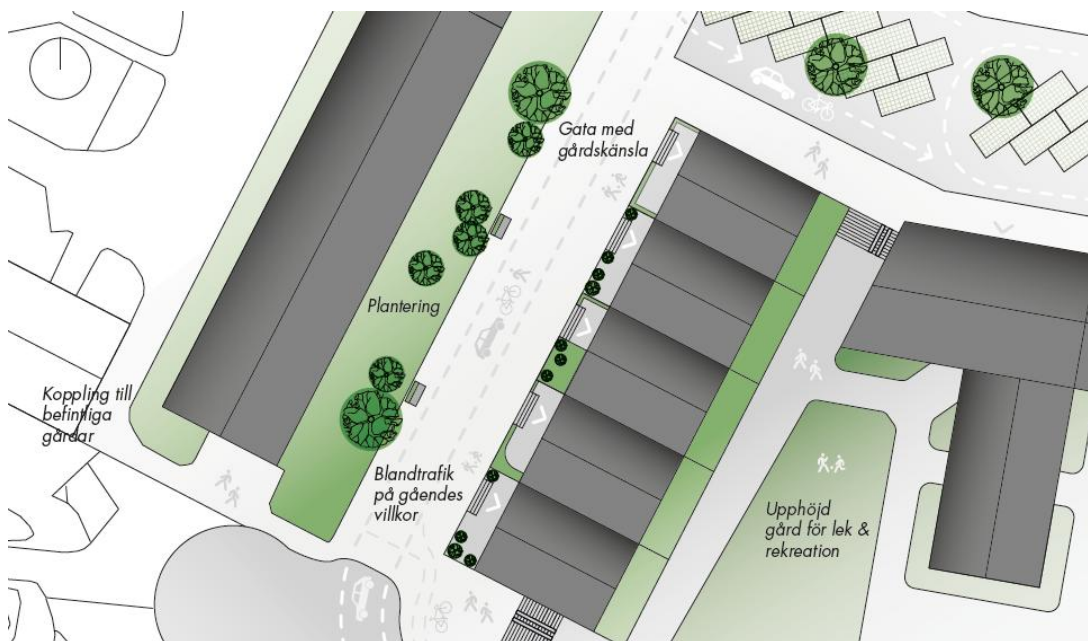
Principskiss för hur radhus möter befintlig bebyggelse. Bild: OkiDoki arkitekter
