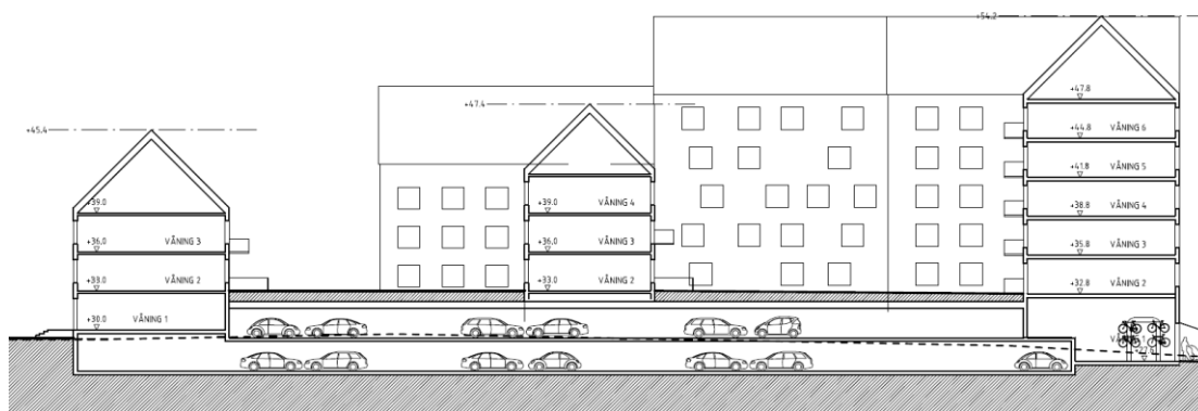
Principsektion där parkeringsgaraget i ett plan är nedgrävt. Streckad linje visar befintlig marknivå. Bild: OkiDoki arkitekter
